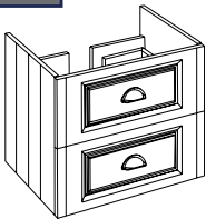
(H) 480mm x (W) 600mm x (D) 445mm
