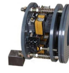
AC EM Disc Brake
