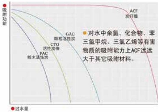
吸附功能对比表 Adsorption Function Comparison Table
