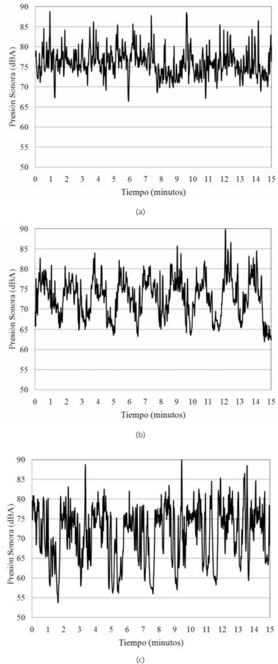
Figura 1. Nivel de presión sonora sin integrar - L_p (segundo a segundo por períodos de 15 minutos): a) Carrera 30; b) Carrera Séptima; c) Avenida Circunvalar.
