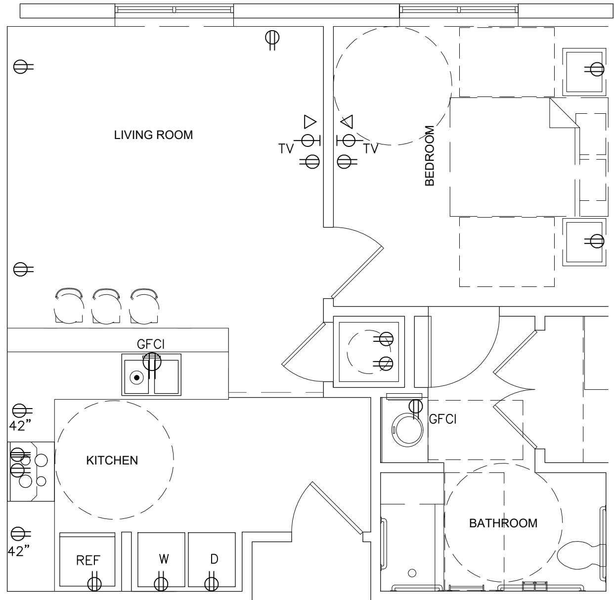
APT D (DAMANSARA) (638 SF)
