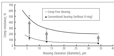
Fig. 2 Creep limit load test (example: 6204)
