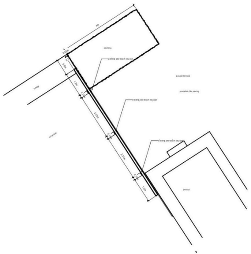
4 Jacuzzi Pergola Plan View Scale: 1:50
