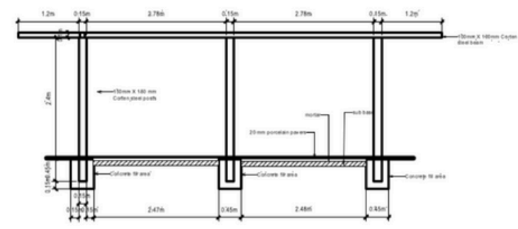
2 Three Post Pergola Scale: 1:50
