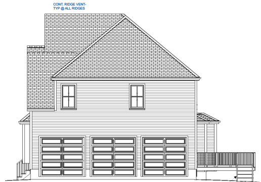
Right Elevation scale: 1/4" = 1'
