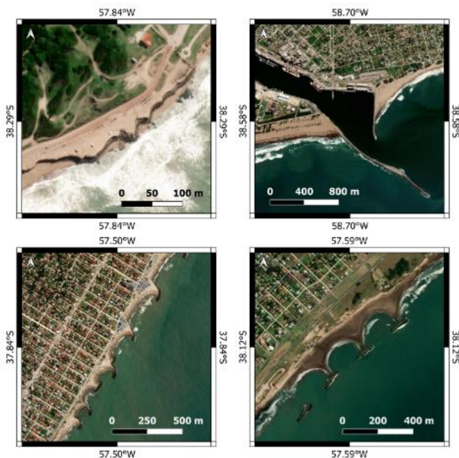
Figura 55. Defensas costeras identificadas en el litoral bonaerense: protecciones paralelas de acantilados vivos Miramar (superior izquierda), obras de abrigo del Puerto Quequén (superior derecha), escolleras en la localidad de Santa Clara del Mar (inferior izquierda), rompeolas vinculados y desvinculados de la costa en Barrio Los Acantilados (inferior derecha). Fuente: Elaboración propia.
