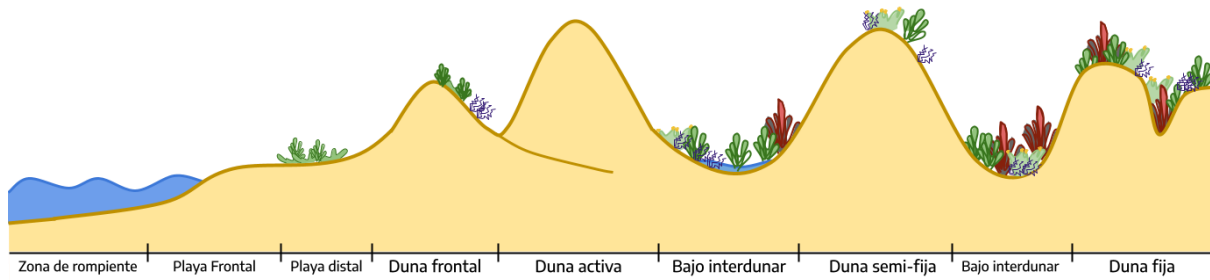
Figura 51. Perfil típico del sistema playa-duna en costas blandas.
