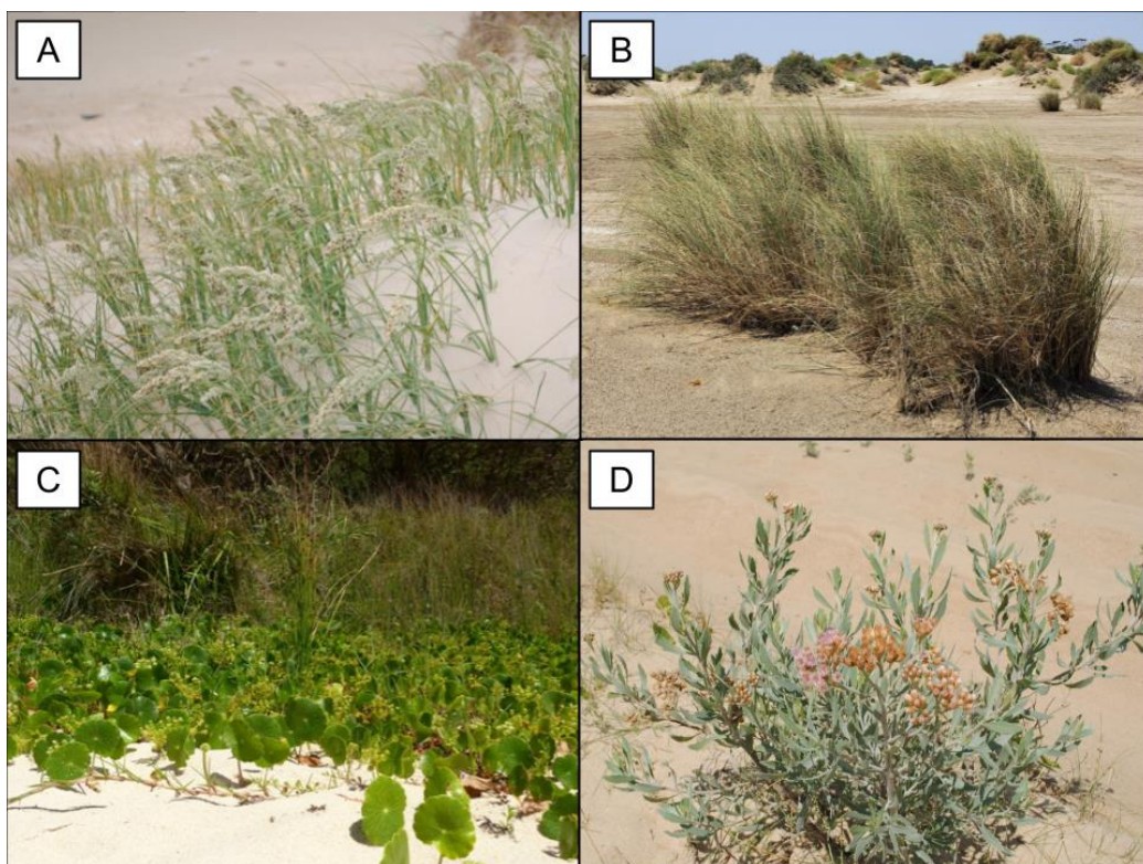
Figura 73. Ejemplos de vegetación nativa de las dunas bonaerenses: Panicum racemosum (A), Spartina ciliata (B); Hydrocotyle bonariensis (C); Tessaria absinthoides (D). Fuente: Isla et al. (2023)
