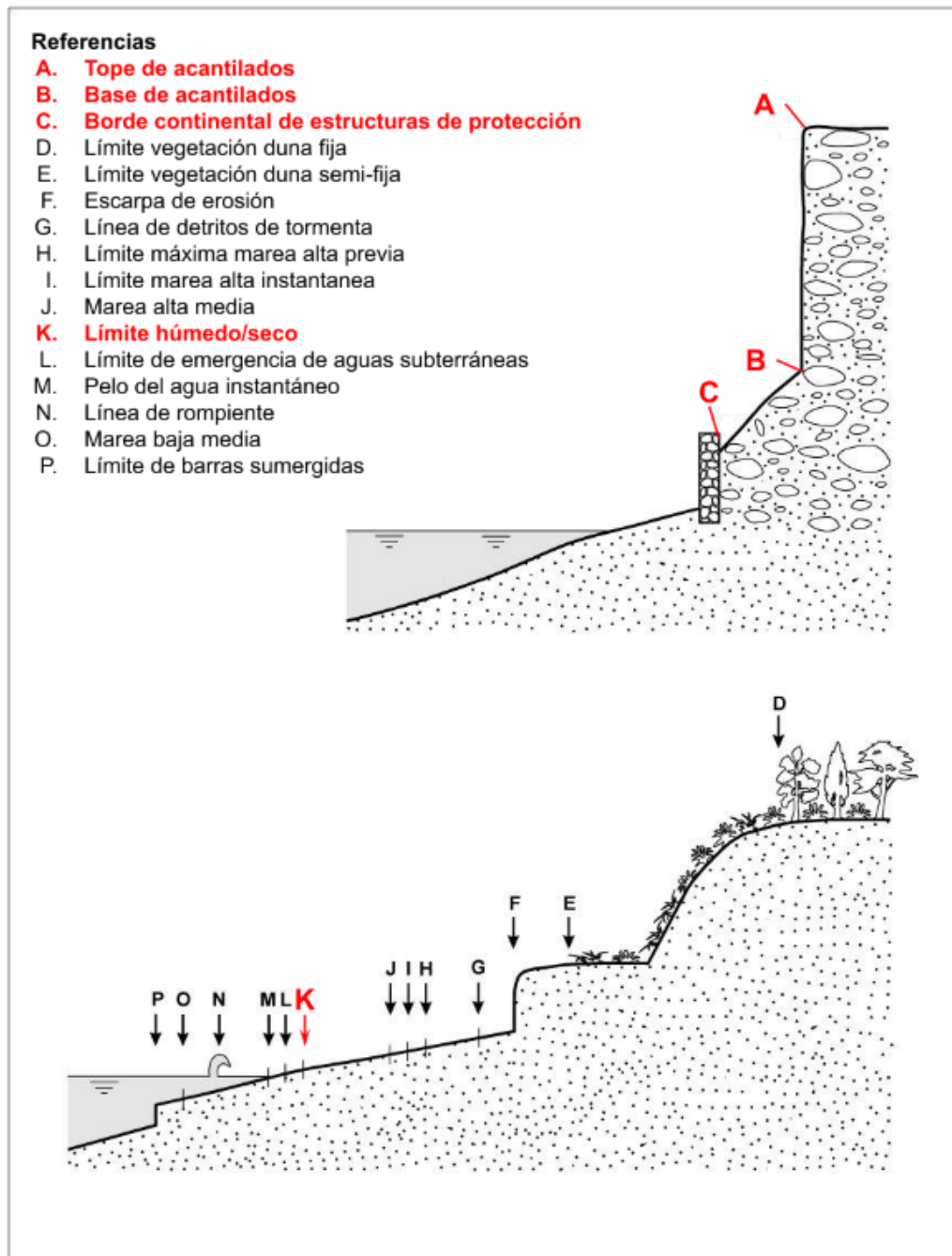
Figura 53. Proxys utilizados para la delimitación posicional de la línea de costa. En rojo se destacan los utilizados en este capítulo. Fuente: Esquema adaptado a partir de Boak and Turner (2005).
