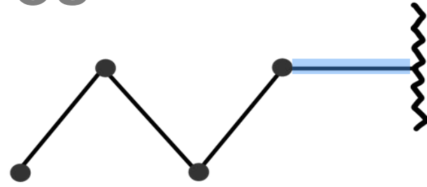
butil
