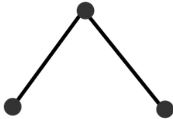
propano
