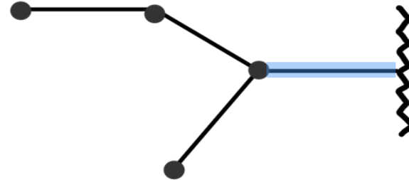
secbutil
