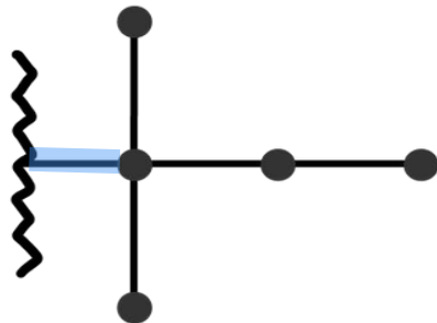
terpentil
