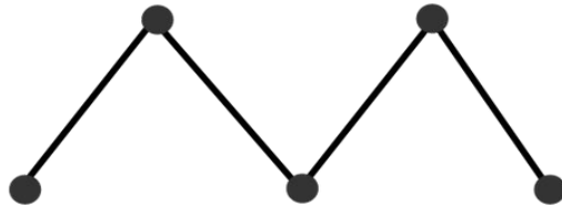
pentano
