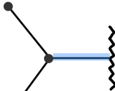
isopropil
