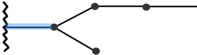
secpentil
