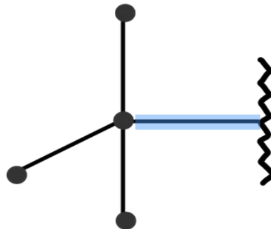
tercbutil
