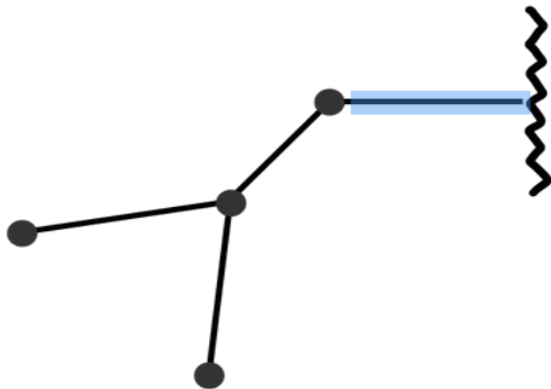
isobutil
