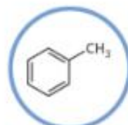
TOLUENE Methylbenzene C_7H_8
