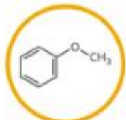
ANISOLE Methoxybenzene C_6H_5OCH_3
