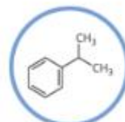
CUMENE Isopropylbenzene C_9H_{12}
