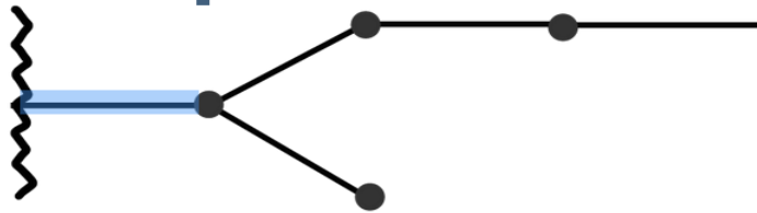
pentano
