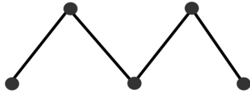
pentano
