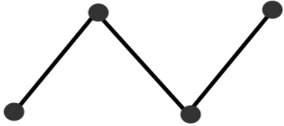
butano
