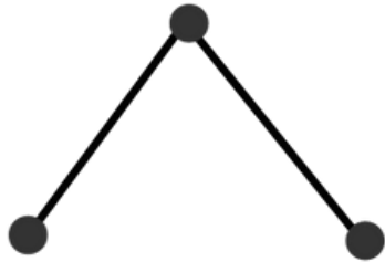
propano
