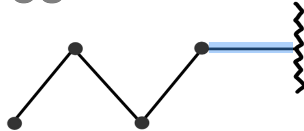
butil
