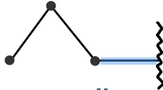
propil
