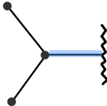
isopropil
