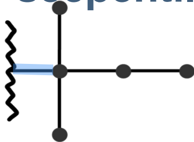
terpentil
