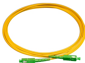
Cordão Óptico Simplex SC APC x SC APC 2.0MM x 1,5M Monomodo
