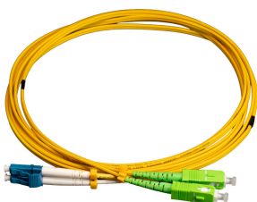
Cordão Óptico Duplex LC UPC x SC APC 2.0MM x 1,5M Monomodo
