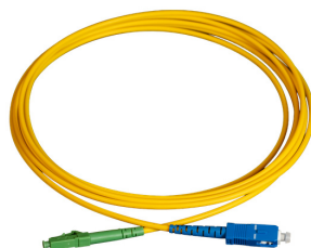
Cordão Óptico Simplex SC UPC x LC APC 2.0MM x 1,5M Monomodo
