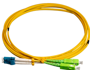
Cordão Óptico Duplex LC UPC x SC APC 2.0MM x 5M Monomodo
