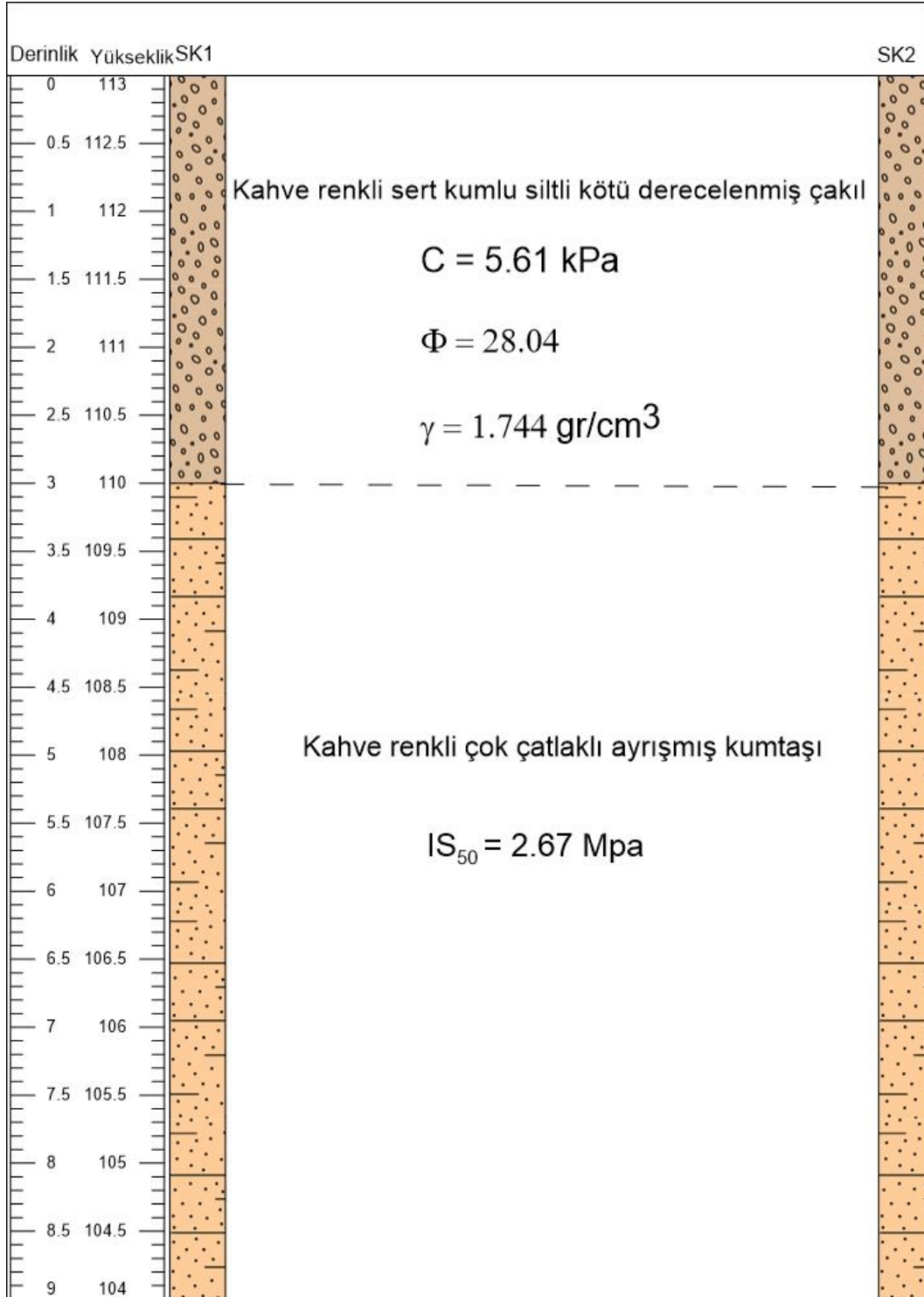
Şekil 2 İdealize Zemin Profili
