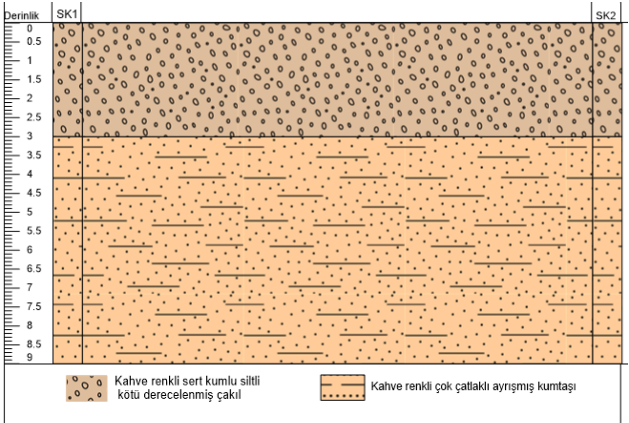
Şekil 9 Jeolojik Kesit
