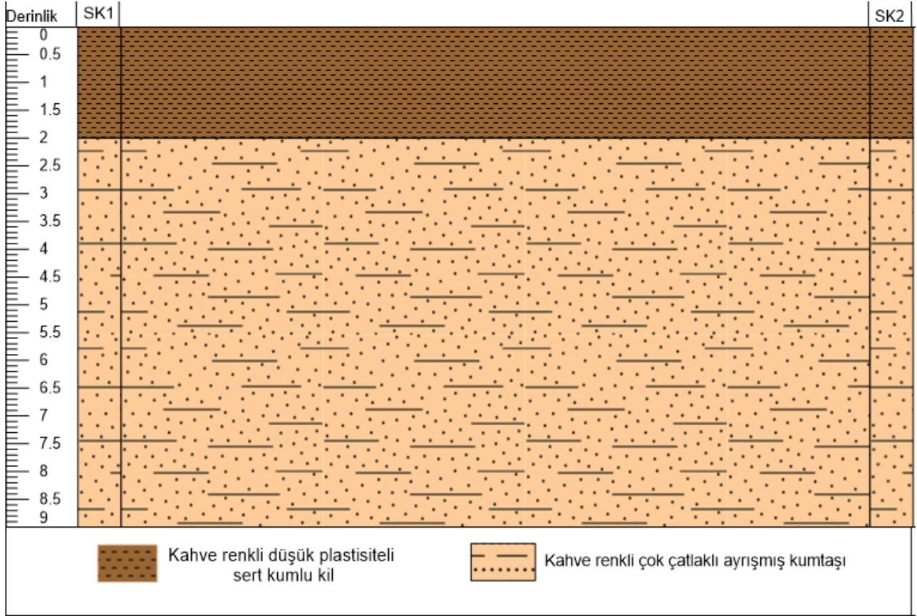
Şekil 9 Jeolojik Kesit
