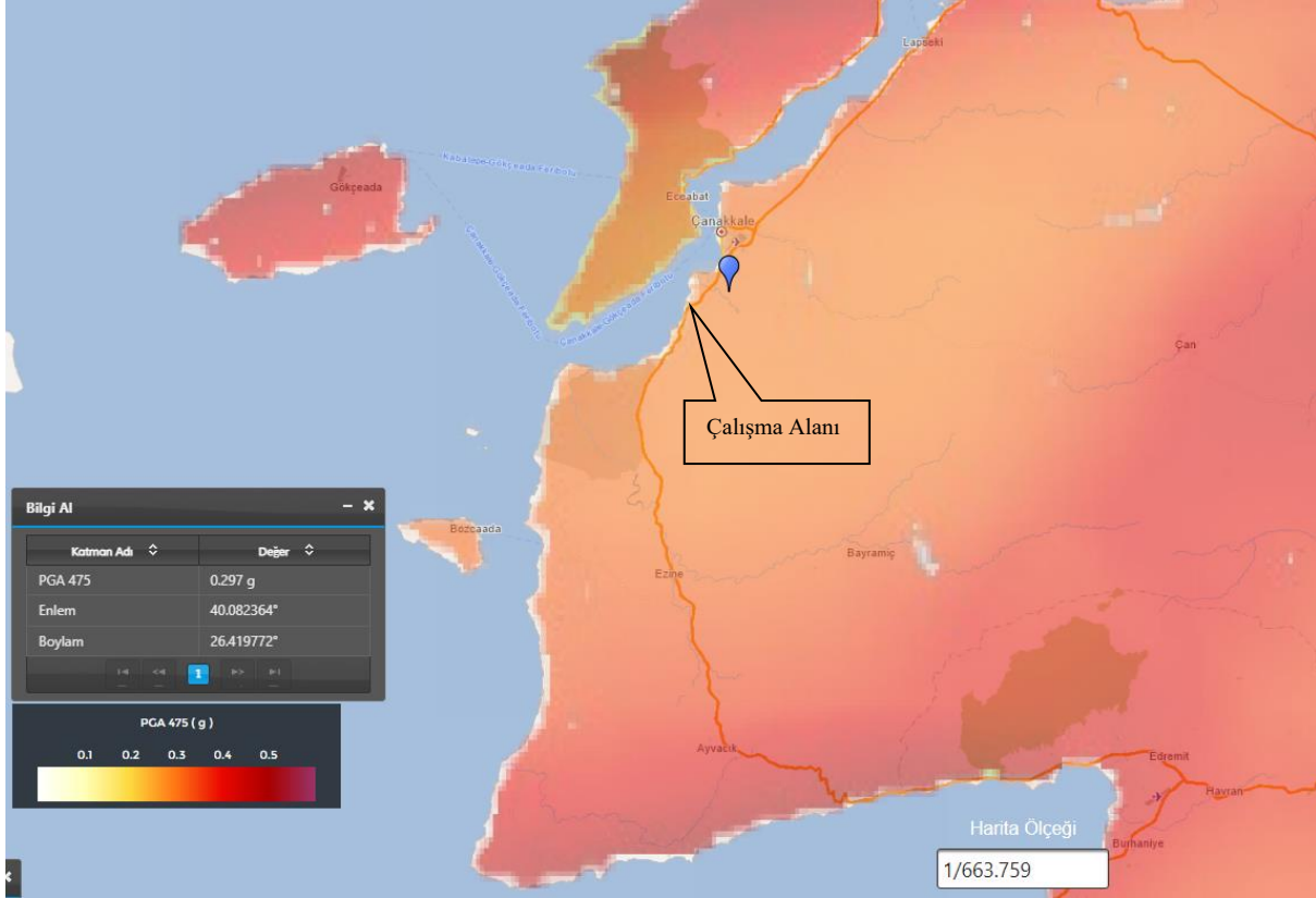
Şekil 3: Çanakkale bölgesi deprem tehlike haritası
