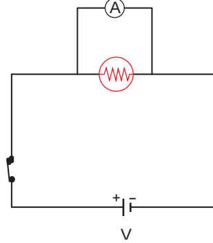
Şekil 1.11: Basit elektrik devresine paralel bağlı ampermetre
