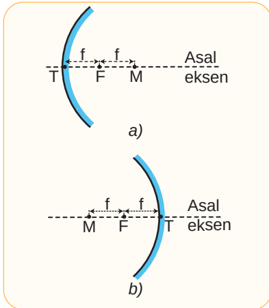
Şekil 4.21: a) Çukur aynanın asal eksen üzerindeki tepe (T), odak (F) ve merkez (M) noktaları b) Tümsek aynanın asal eksen üzerindeki tepe (T), odak (F) ve merkez (M) noktaları
