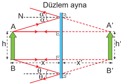
Şekil 4.17: Düzlem aynada bir cismin görüntüsü
