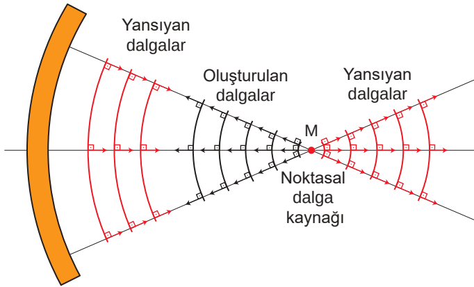
Şekil 3.35: Eğrilik merkezine yerleştirilen noktasal dalga kaynağından çıkan dalgaların parabolik engelden yansıması
