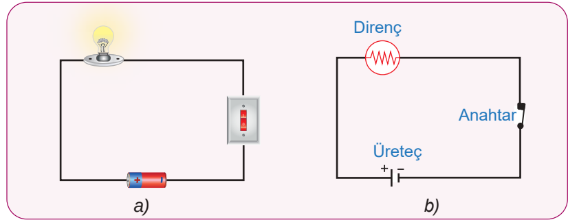
Şekil 1.7: a) Basit elektrik devresi b) Basit elektrik devresinin şematik gösterimi
