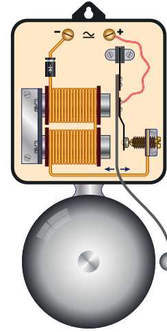
Görsel 1.20: Kapı zilin yapısı
