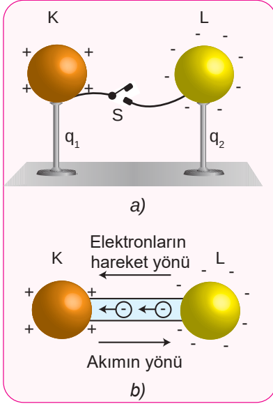
Şekil 1.2: a) Yük miktarları farklı özdeş iletken küreler b) Anahtar kapatıldığında telden geçen akımın ve elektronların hareket yönü
