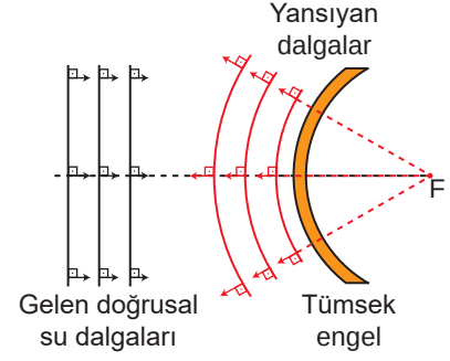
Şekil 3.32: Doğrusal su dalgalarının tümsek engelden yansımasının üstten görünümü
