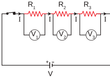
Şekil 1.16: Seri bağlı dirençlerin şematik gösterimi
