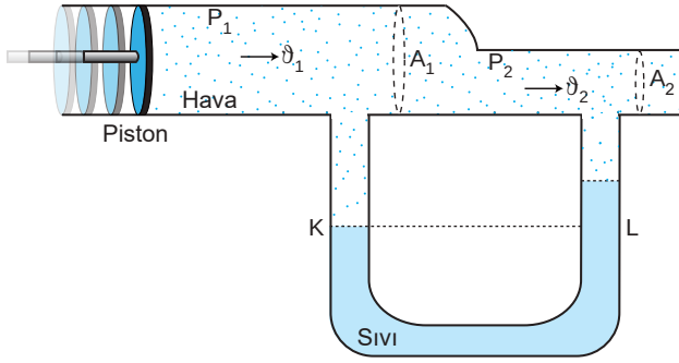
Şekil 2.32: Kesit alanı daralan boru
