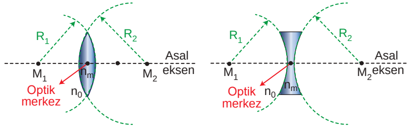
Şekil 4.42: Merceklerin eğrilik yarıçapları ve odak noktaları
