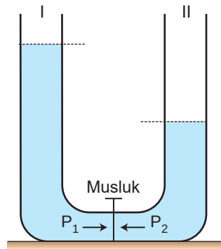
Şekil 2.12: Sıvı seviyeleri farklı bileşik kap
