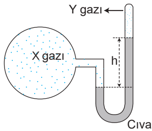
Şekil 2.29: Borusunda gaz bulunan kapalı uçlu manometre
