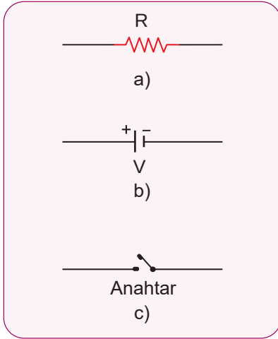
Şekil 1.6: Basit bir elektrik devresinde kullanılan devre elemanlarının şematik gösterimi: a) Direnç, b) Üreteç, c) Anahtar
