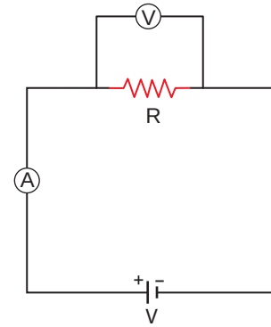
Şekil 1.22: Voltmetre ve ampermetre bağlı basit elektrik devresi
