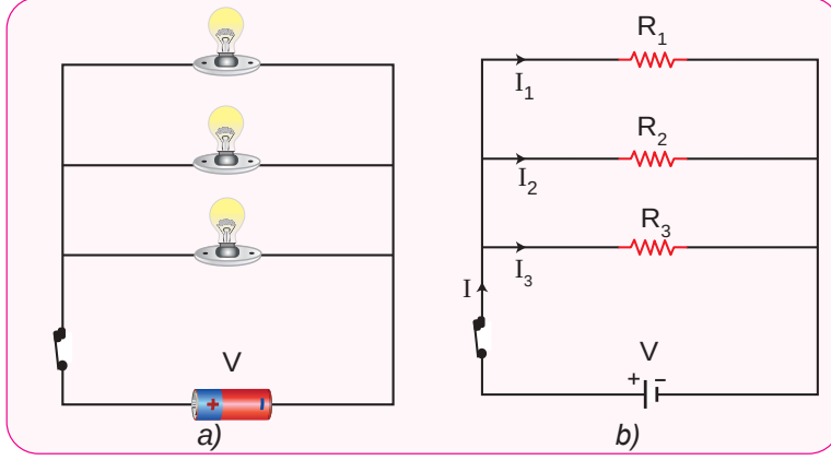
Şekil 1.17: a) Paralel bağlı lambalar b) Paralel bağlı dirençlerin şematik gösterimi
