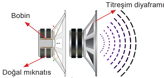
Görsel 1.19: Hoparlörün yapısı
