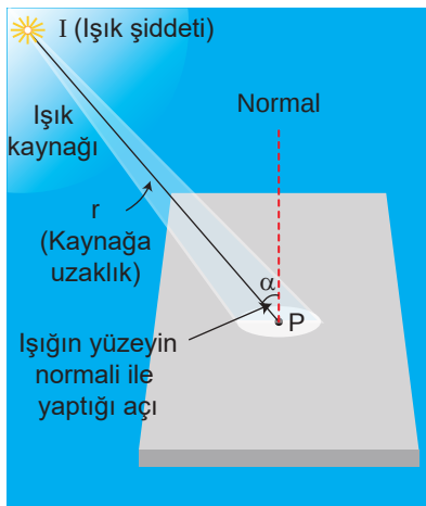
Şekil 4.5: P noktası çevresindeki aydınlanma şiddeti
