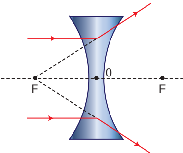
Şekil 4.44: Kalın kenarlı merceğin odak noktası
