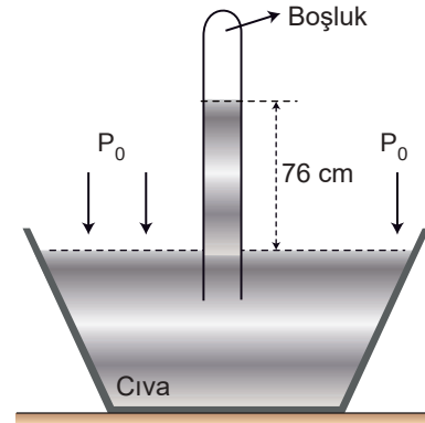
Şekil 2.19: Torricelli deneyi (Barometre)
