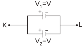
Şekil 1.21: Paralel bağlı özdeş pillerin şematik gösterimi
