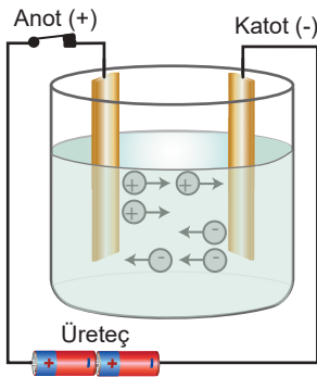
Şekil 1.4: Sıvılarda artı (+) ve eksi (-) iyonların oluşturduğu elektrik akımı
