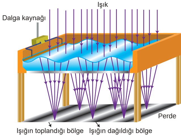
Şekil 3.25: Dalga leğeninin altına yerleştirilen perdenin üzerinde oluşan aydınlık ve karanlık bölgeler
