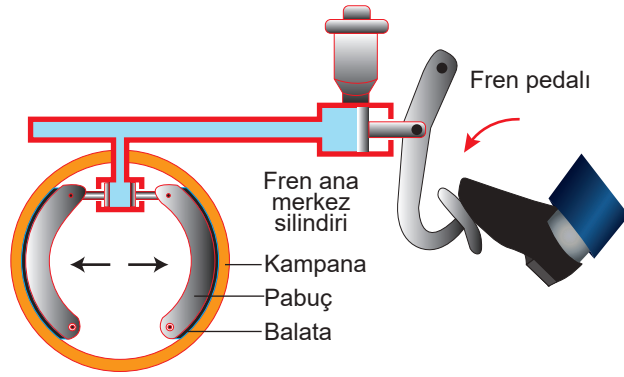
Şekil 2.14: Hidrolik fren sistemi
