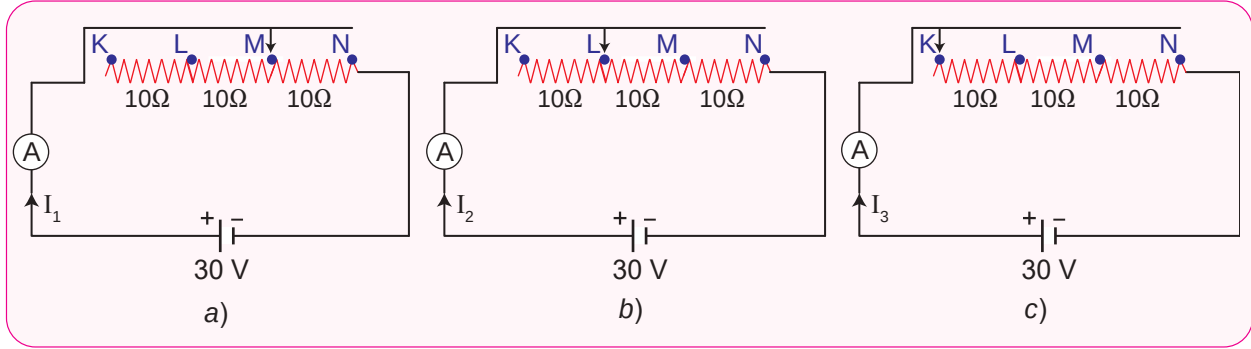
Şekil 1.14: a, b, c) Reostalı elektrik devresinde sürgü hareketinin incelenmesi
