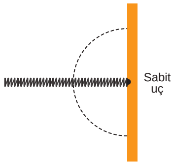
Şekil 3.22: Sabit uçta yansıma sırasında yıkıcı girişim
