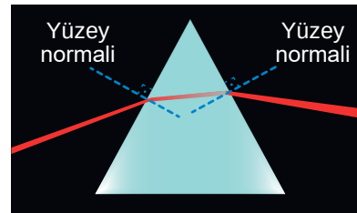
Şekil 4.49: Kırmızı LASER ışığının cam prizmadan geçişi
