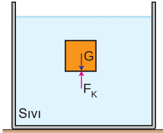
Şekil 2.37: Sıvıda askıda kalan cisim
