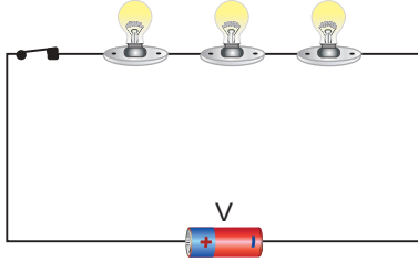
Şekil 1.15: Seri bağlı lambalar
