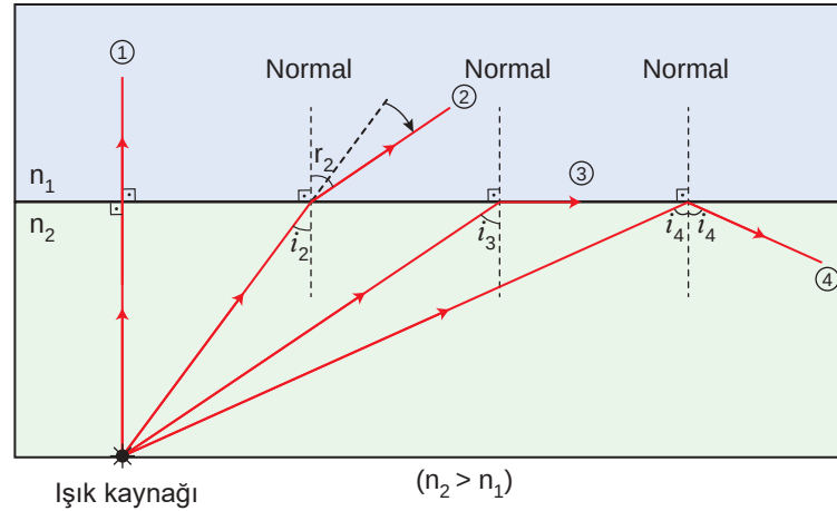
Şekil 4.28: Kırılma indisi büyük olan ortamdan kırılma indisi küçük olan ortama gönderilen ışınların izlediği yollar
