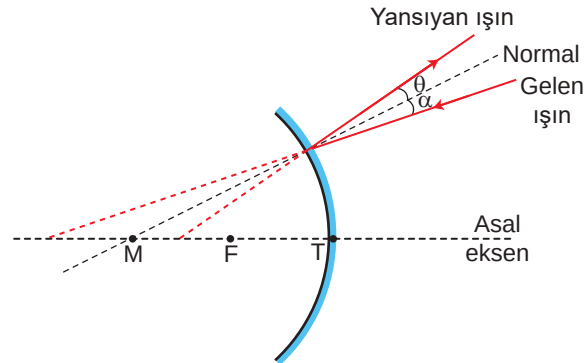
Şekil 4.23: Tümsek aynada ışının yansıması
