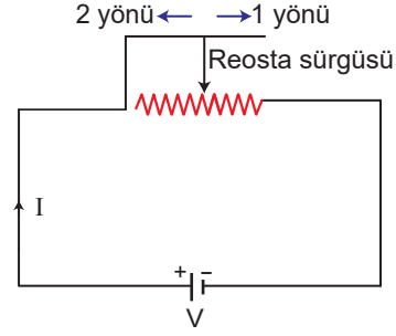
Şekil 1.13: Reostalı elektrik devresi
