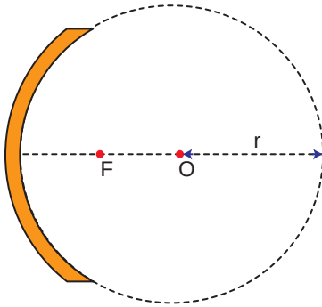
Şekil 3.33: Parabolik engelin merkez ve odak noktası
