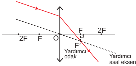
Şekil 4.45: Özel olmayan ışının ince kenarlı mercekte kırılması
