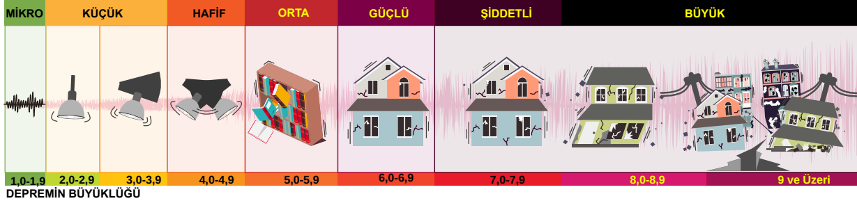
Şekil 3.49: Depremin şiddeti ile büyüklüğü arasındaki ilişki
