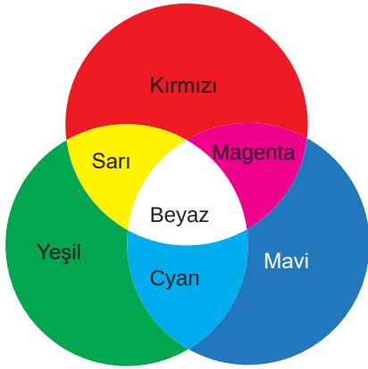
Şekil 4.55: Işık renklerinin karışımı
