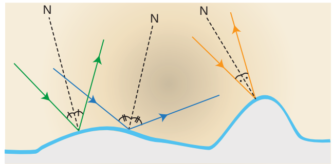
Şekil 4.15: Dağınık yansıma
