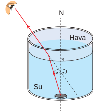
Şekil 4.33: Su içerisindeki metal paranın görülmesi
