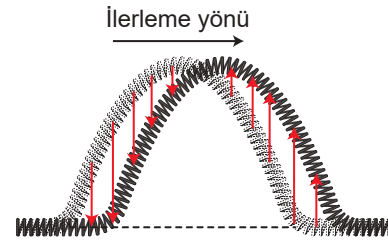
Şekil 3.14: Atmanın ilerlemesi
