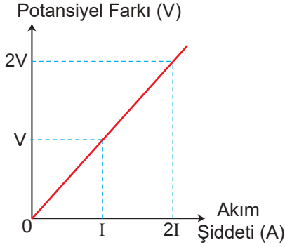
Şekil 1.12: Potansiyel farkı - Akım şiddeti grafiği
