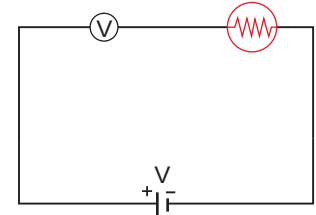
Şekil 1.9: Devre elemanına seri bağlı voltmetre
