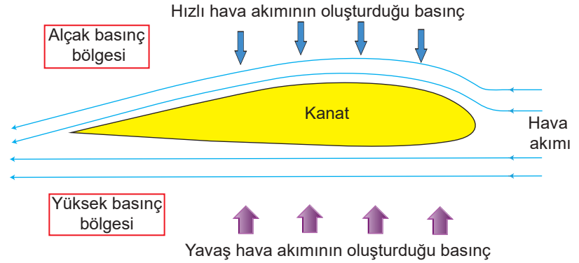
Şekil 2.33: Uçak kanadı kesiti
