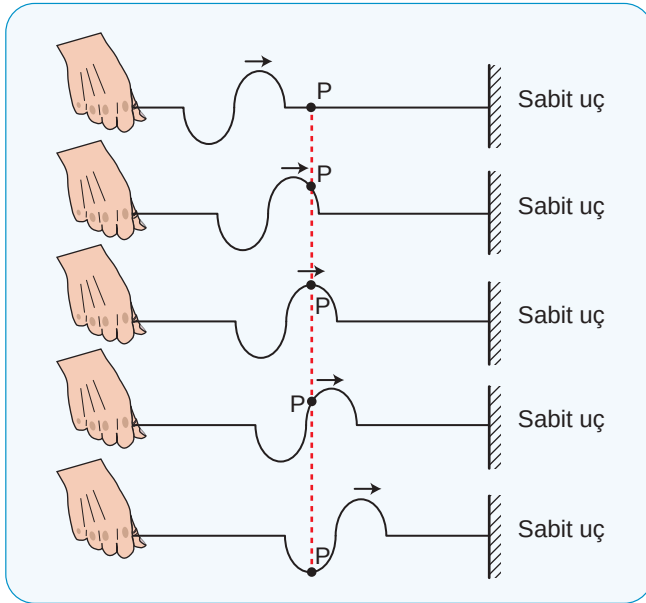
Şekil 3.3: Oluşturulan bir dalgaının ilerlemesi sırasında ortam üzerindeki P noktasının hareketi
