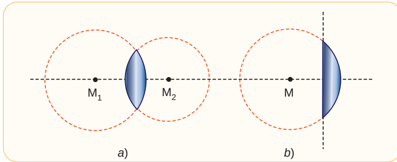
Şekil 4.38: İnce kenarlı mercek örnekleri
