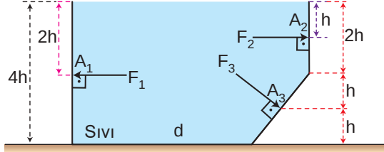
Şekil 2.17: Yan yüzeylere etki eden sıvı basınç kuvveti
