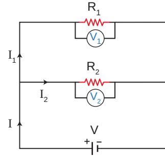
Şekil 1.18: Dirençlerin paralel bağlanmasıyla oluşturulan elektrik devresi
