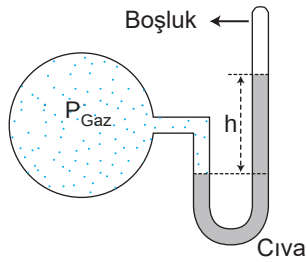
Şekil 2.28: Kapalı uçlu manometre
