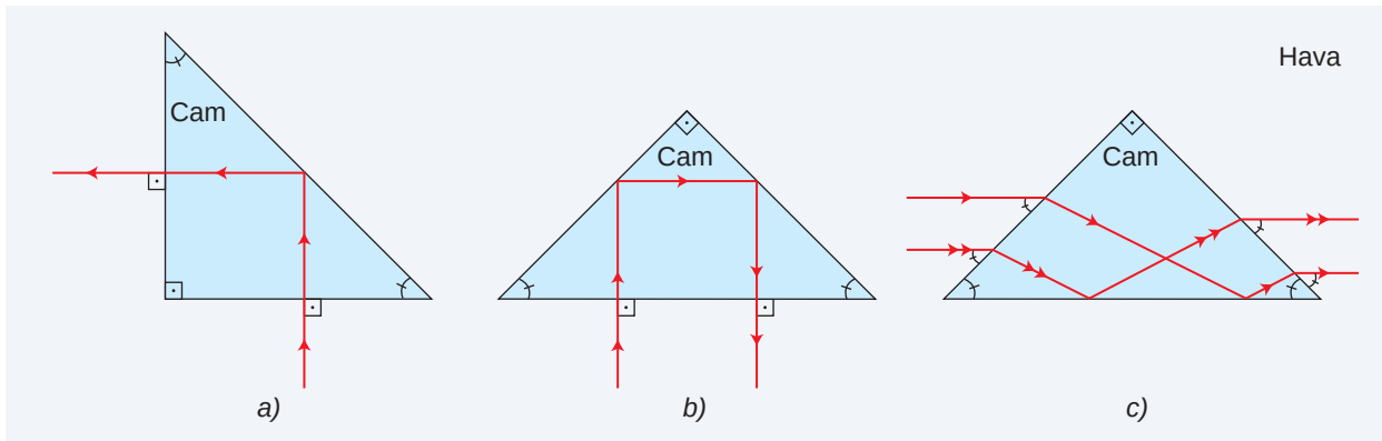
Şekil 4.50: Bazı ışınların tam yansımali prizmalarda kırılması
