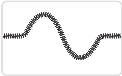
Şekil 3.6: Yay dalgası
