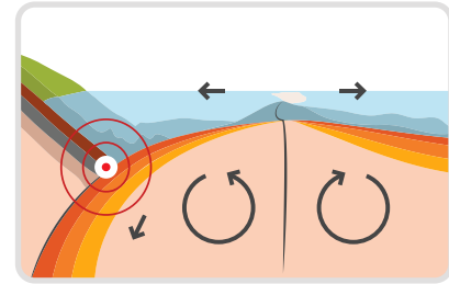
Şekil 3.5: Deprem dalgası
