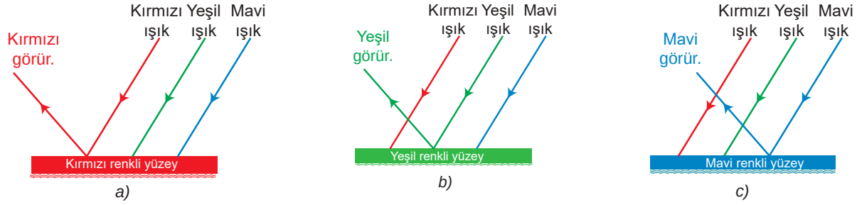
Şekil 4.57: Kırmızı, yeşil ve mavi renkli yüzeylerden güneş ışığının yansımaları
