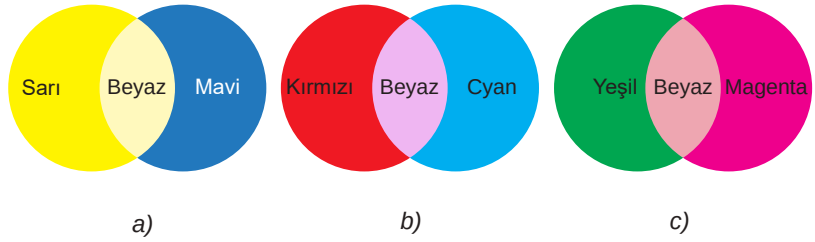
Şekil 4.56: a, b, c) Tamamlayıcı renkler
