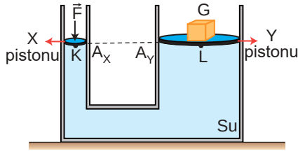
Şekil 2.13: Su cenderesi
