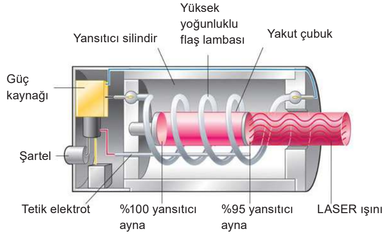
Şekil 6.10: LASER cihazı
