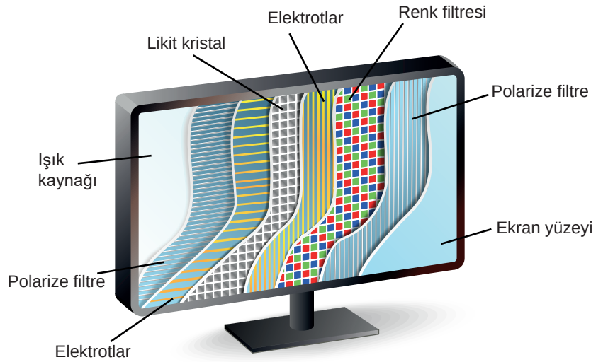
Şekil 6.1: LCD panel yapısı
