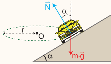
Şekil 1.9: b) Aracın serbest cisim diyagramı
