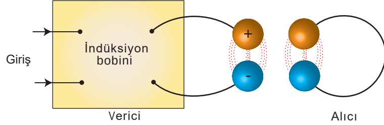
Şekil 5.9: Hertz'in elektromanyetik dalga üretip bu dalgaları algıladığı düzeneğin şematik gösterimi
