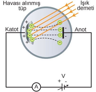
Şekil 5.17: Fotoselli devreye ters bağlanmış üretel
