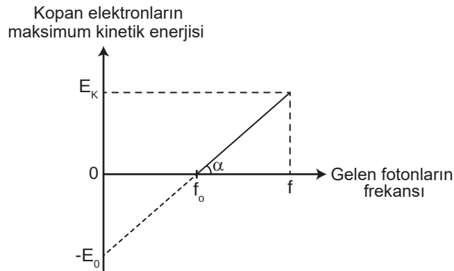
Şekil 5.11: Kopan elektronların kinetik enerjilerinin gelen fotonların frekansına bağlı değişim grafiği
