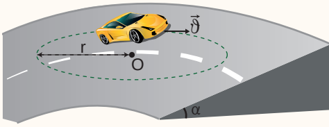
Şekil 1.9: a) Sürtünmesiz eğimli virajda hareket eden araç
