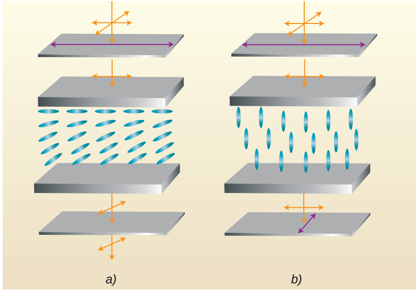
Şekil 6.2: a) Sıvı kristal hücrelerinin gerilimi uygulanmadan önceki duruşları b) Sıvı kristal hücrelerinin gerilimi uygulandıktan sonraki duruşları
