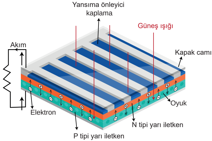
Şekil 6.5: Fotovoltaik dönüşüm sistemi
