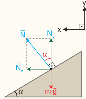
Şekil 1.9: c) Araca etki eden kuvvetlerin x-y eksenindeki bileşenleri
