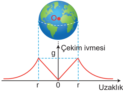
Şekil 1.25: Çekim ivmesinin Dünya'nın merkezine olan uzaklığına bağlı değişim grafiği
