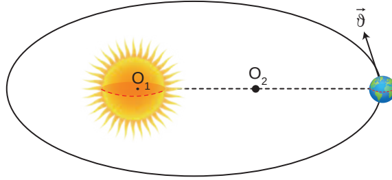
Şekil 1.26: Dünya'nın Güneş etrafındaki eliptik yörüngesi ( O_1 ve O_2 elipsin odaklarıdır.)
