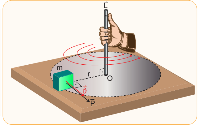
Şekil 1.19: Çembersel hareket yapan bir cismin sağ el kuralıyla açısal momentumunun yönünün gösterilmesi
