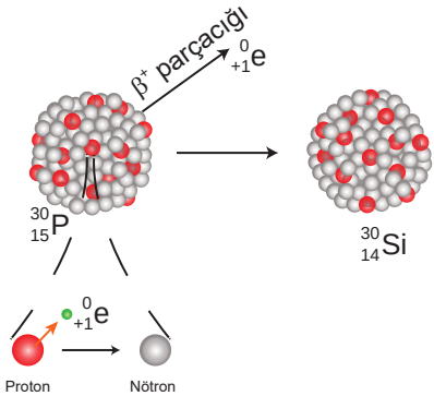
Şekil 4.26: \beta^+ bozunumu
