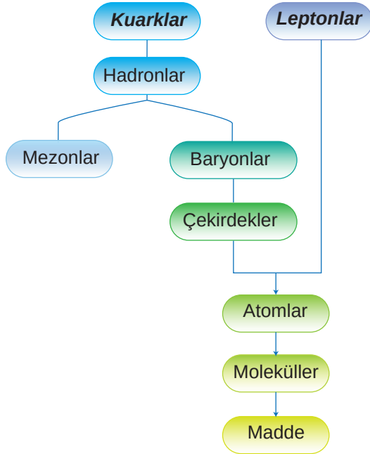
Şekil 4.21: Madde oluşum süreci
