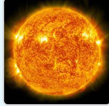
Görsel 5.3: Güneş'in ışıması
