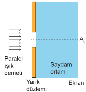
Şekil 3.21: Yarık düzlemi ile ekran arasında havadan daha yoğun saydam ortam bulunması
