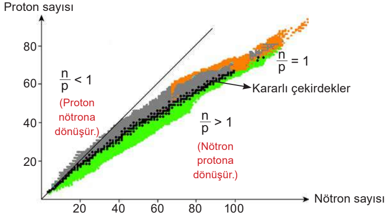
Şekil 4.23: Elementlerin proton ve nötron sayılarının değişimine bağlı olarak nükleer kararsızlık eğrisi
