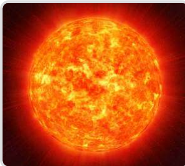
Görsel 6.21: Güneş
