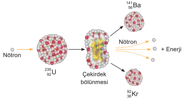
Şekil 4.28: Filyon tepkimesi
