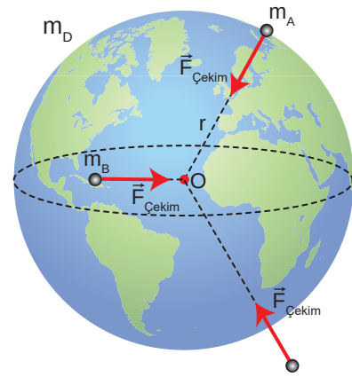
Şekil 1.24: Dünya yüzeyindeki ( m_A ), içindeki ( m_B ) ve dışındaki ( m_C ) herhangi bir cisme uygulanan yer çekimi kuvveti
