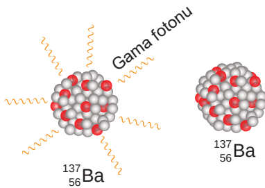
Şekil 4.27: γ bozunumu
