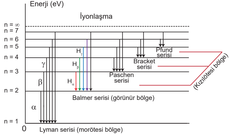
Şekil 4.11: Uyarılmış bir hidrojen atomunda elektronların temel hâle dönerken oluşturduğu seriler
