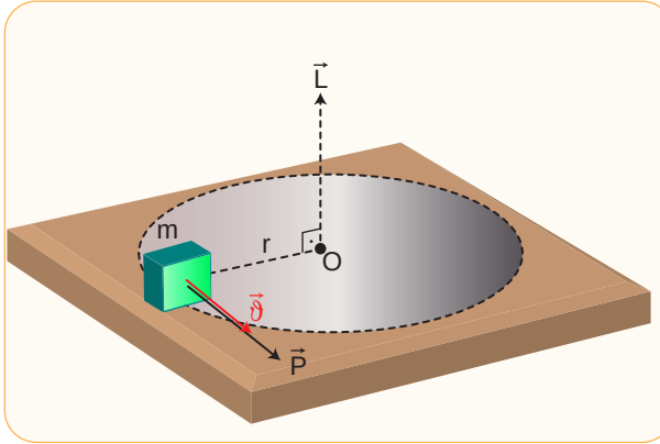
Şekil 1.18: Çembersel hareket yapan cisim
