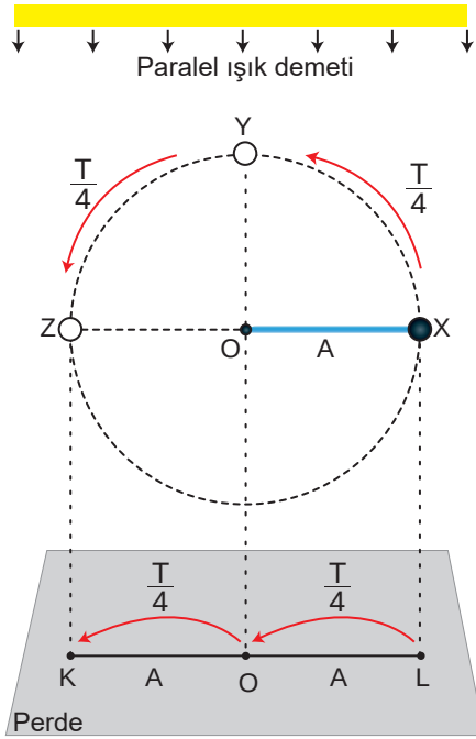
Şekil 2.6: Düzgün çembersel hareketin yatay eksendeki iz düşümü
