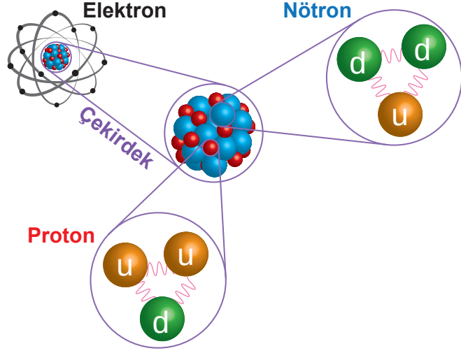
Şekil 4.22: Atomun yapısında bulunan temel parçacıklar
