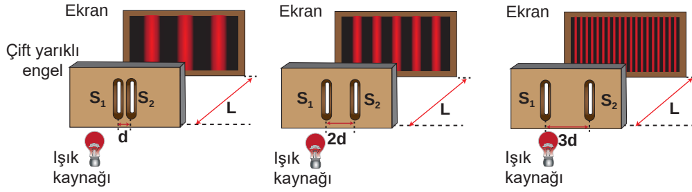
Şekil 3.10: Yarıklar arası uzaklığı farklı olan çift yarıktaki girişim deneyinde kırmızı ışığın girişim deseni
