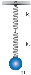
Şekil 2.17: Seri bağlı yaylar
