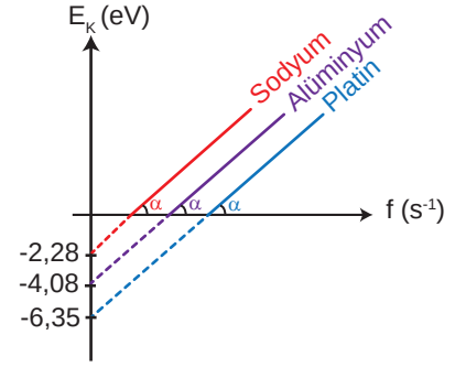
Şekil 5.12: Farklı metallerden koparılan elektronların kinetik enerjilerinin gelen fotonların frekansına bağlı değişim grafiği
