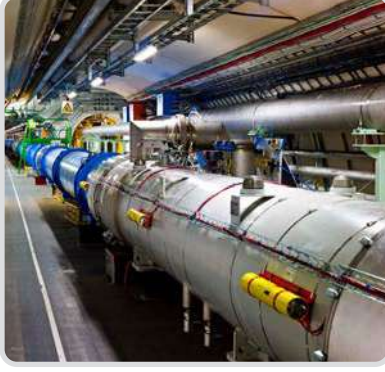
Görsel 6.26: Parçacık hızlandırıcılarda kullanılan süper iletken bobin
