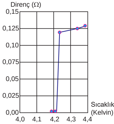
Şekil 6.6: Cıvanın direncinin sıcaklığa bağlı değişim grafiği
