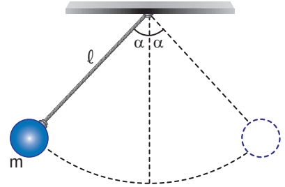
Şekil 2.20: Basit sarkaç ( \alpha < 10^\circ )
