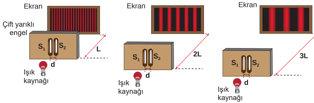
Şekil 3.11: Yarık düzlemi ile ekran arası uzaklığı farklı olan çift yarıktaki girişim deneyinde kırmızı ışığın girişim deseni
