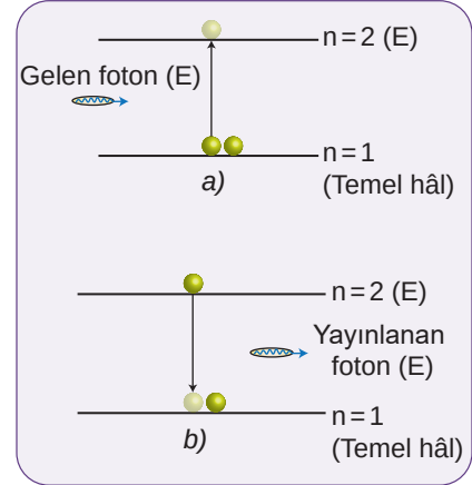
Şekil 6.8: a, b) Kendiliğinden emisyon
