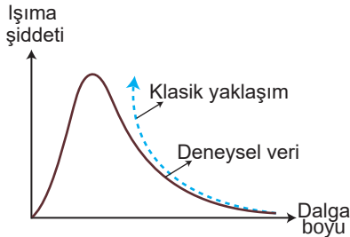
Şekil 5.8: Farklı sıcaklıklar için siyah cismin ışıma şiddetinin ışımanın dalga boyuna bağlı değişim grafiğinin klasik yaklaşımla karşılaştırılması
