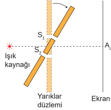
Şekil 3.15: Yarıklık düzleminin döndürülmesi
