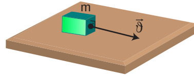
Şekil 1.13: Öteleme hareketi yapan cisim
