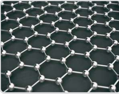
Görsel 6.33: Grafen
