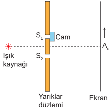
Şekil 3.16: S_1 yarığı önüne cam yerleştirildiğinde merkezî aydınlık saçığının kayma yönü
