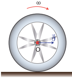
Şekil 1.14: Dönerek ötelenen tekerlek
