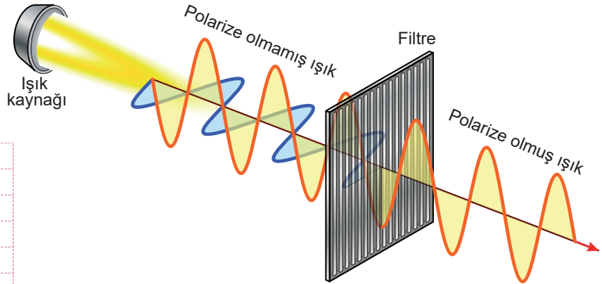
Şekil 3.32: Işığın polarizasyonu
