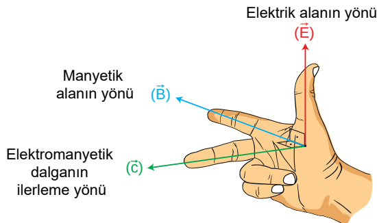
Şekil 3.31: Sağ el kuralı
