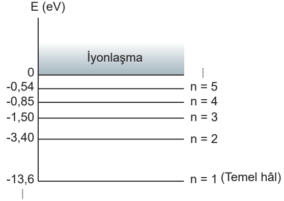
Şekil 4.8: Hidrojen atomunun enerji seviyeleri
