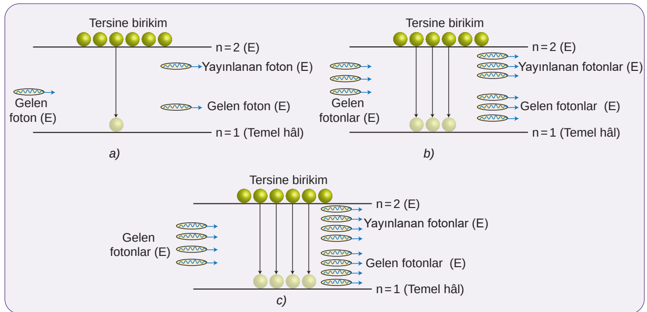
Şekil 6.9: a, b, c) LASER ışığının uyarılmış emisyon yöntemiyle elde edilmesi
