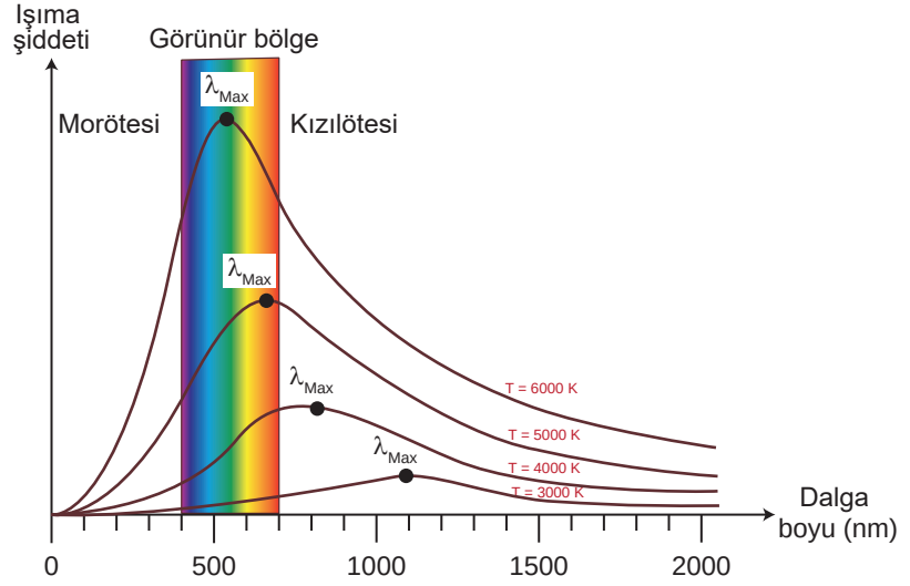
Şekil 5.7: Farklı sıcaklıklar için siyah cismin ışıma şiddetinin ışımanın dalga boyuna bağlı değişim grafiği
