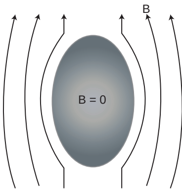
Şekil 6.7: Süper iletken maddenin manyetik alanı dışlaması
