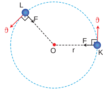
Şekil 1.1: Çembersel hareket yapan cisim
