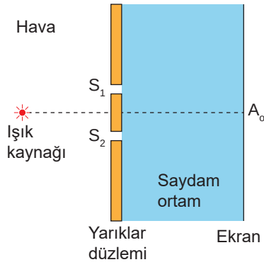
Şekil 3.14: Yarıklık düzlemiyle ekran arasına saydam ortam konulması
