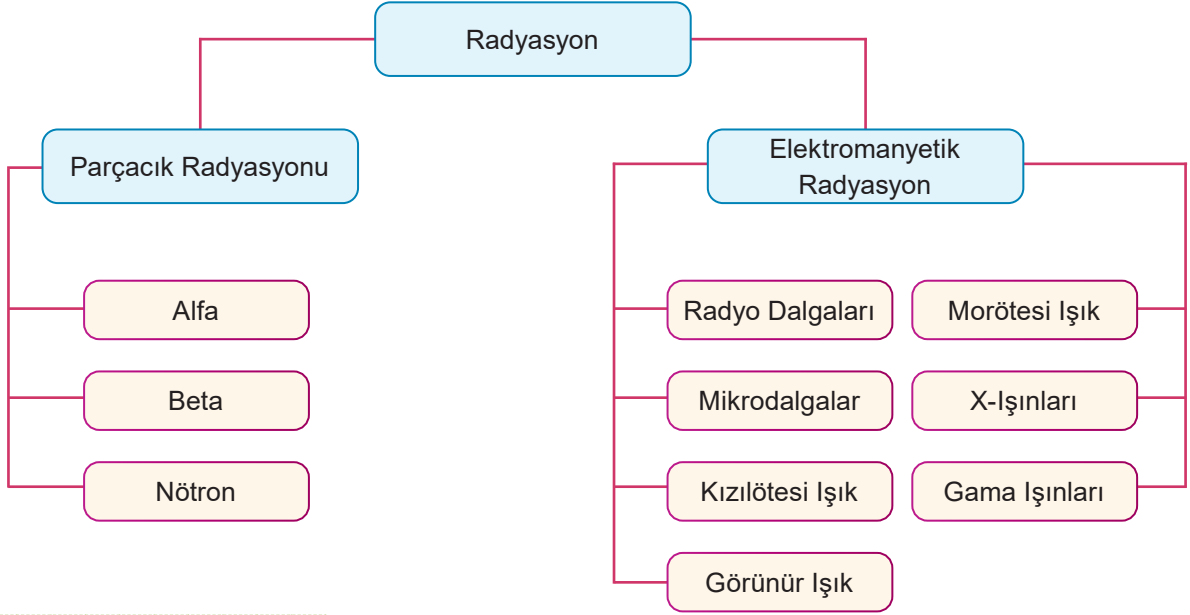
Şekil 4.29: Radyasyon çeşitleri
