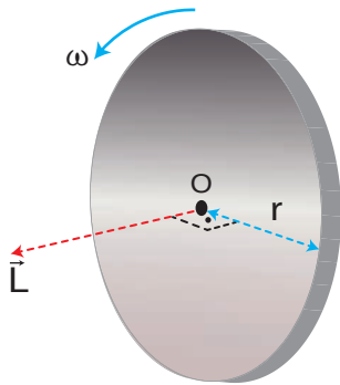
Şekil 1.20: Dönen bir dairesel levhanın açısal momentumu
