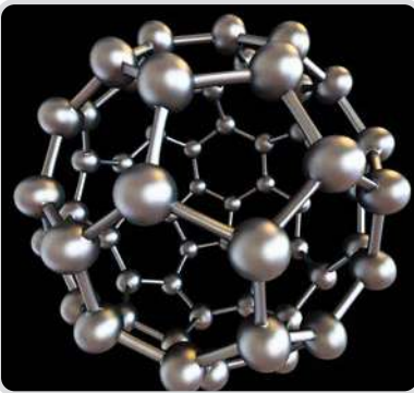
Görsel 6.36: Fulleren
