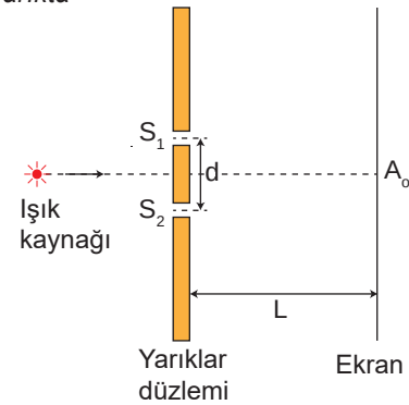
Şekil 3.12: Işık kaynağının yarık düzlemine yaklaştırılması
