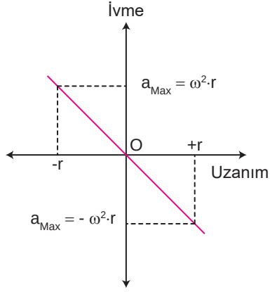
Şekil 2.13: Basit harmonik hareket yapan cismin ivme-uzanım grafiği
