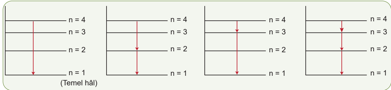
Şekil 4.10: Elektronun temel hâlde farklı geçişleri
