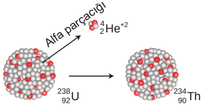
Şekil 4.24: Alfa (α) bozunumu
