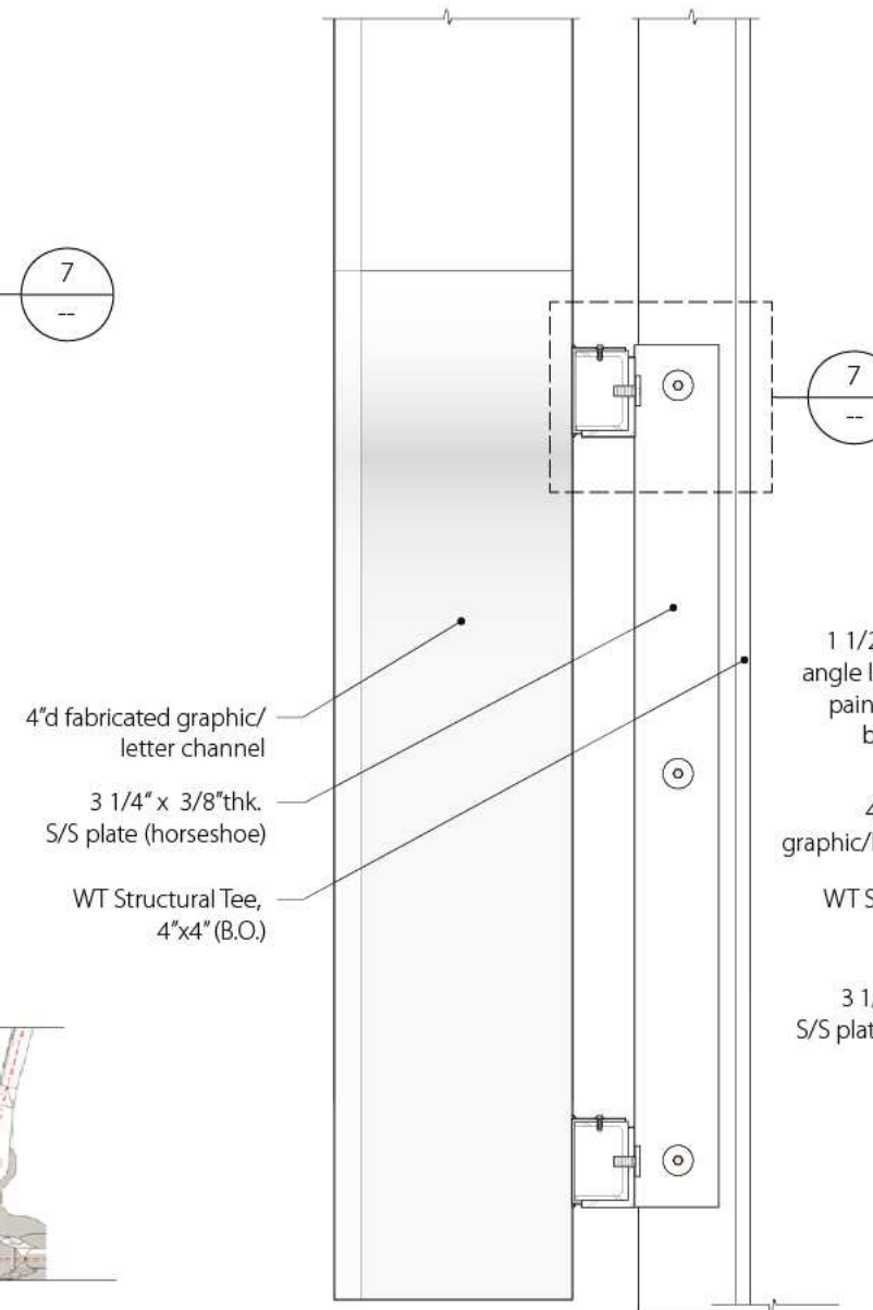
3 END VIEW, Logotype Scale: 1 1/2" = 1'-0"
