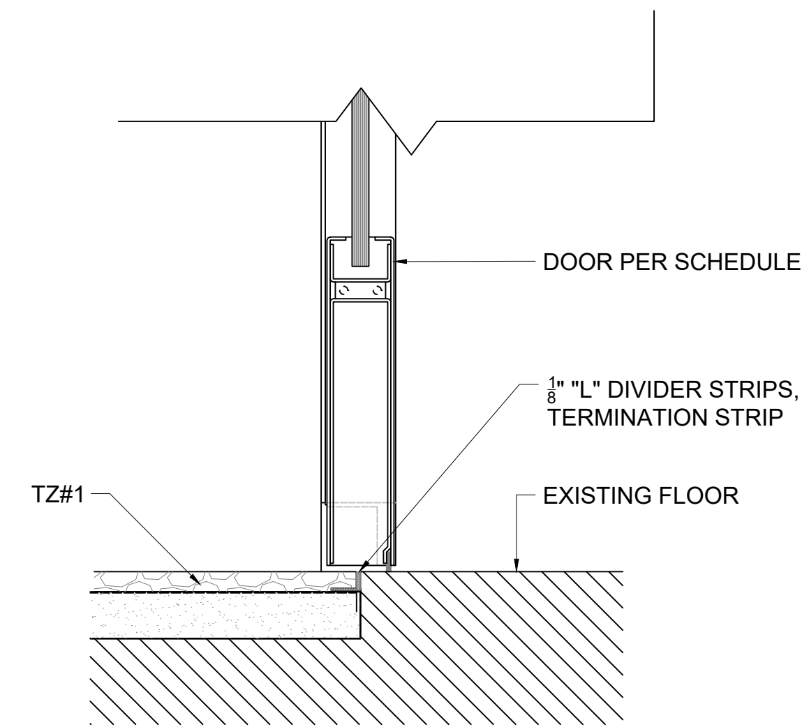
#2—THRESHOLD DETAIL DOOR 3
