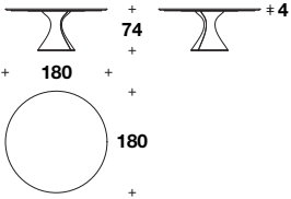
Round table: VTB (24) - VTB (24V) L-D: Ø 180 (Ø 71") H: 74 (29") THK: 4 (1 9/16")
