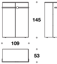
Cabinet: VMB (26) L: 109 (43") D: 53 (21") H: 145 (57")
