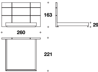
Bed for mattress 195x205 (76 2/3x80 2/3"): GRI (KUSA)
