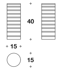
VASE: VBU (06) L-D: Ø 15 (Ø 6") H: 40 (15 3/4")
