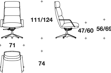
HIGH OFFICE ARMCHAIR: SBG (08)
