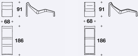
DORMEUSE: ING (CL)
