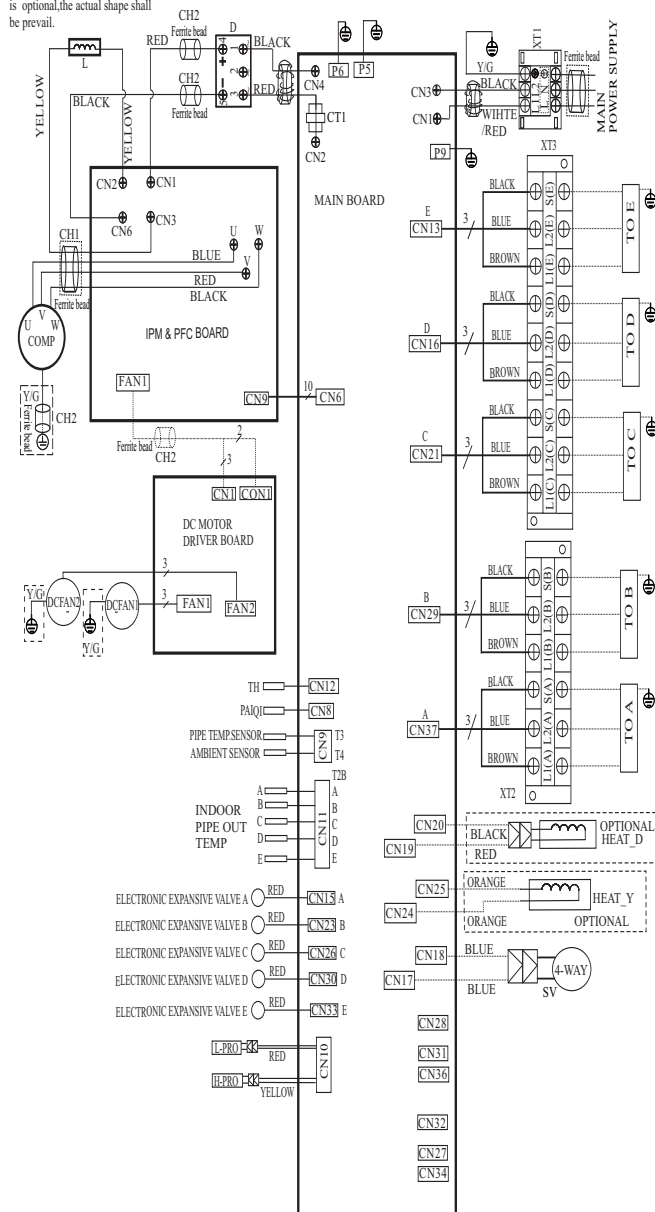
Fig. 14 — Wiring Diagrams 48K — 5 Zone Max
