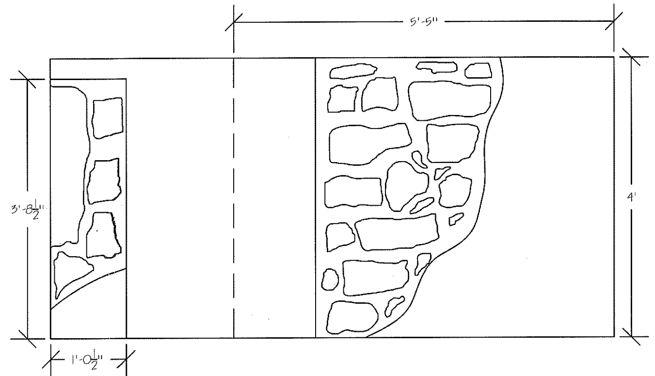
Wall D SL Pivot Wall Scale: 3/4" = 1'-0"
