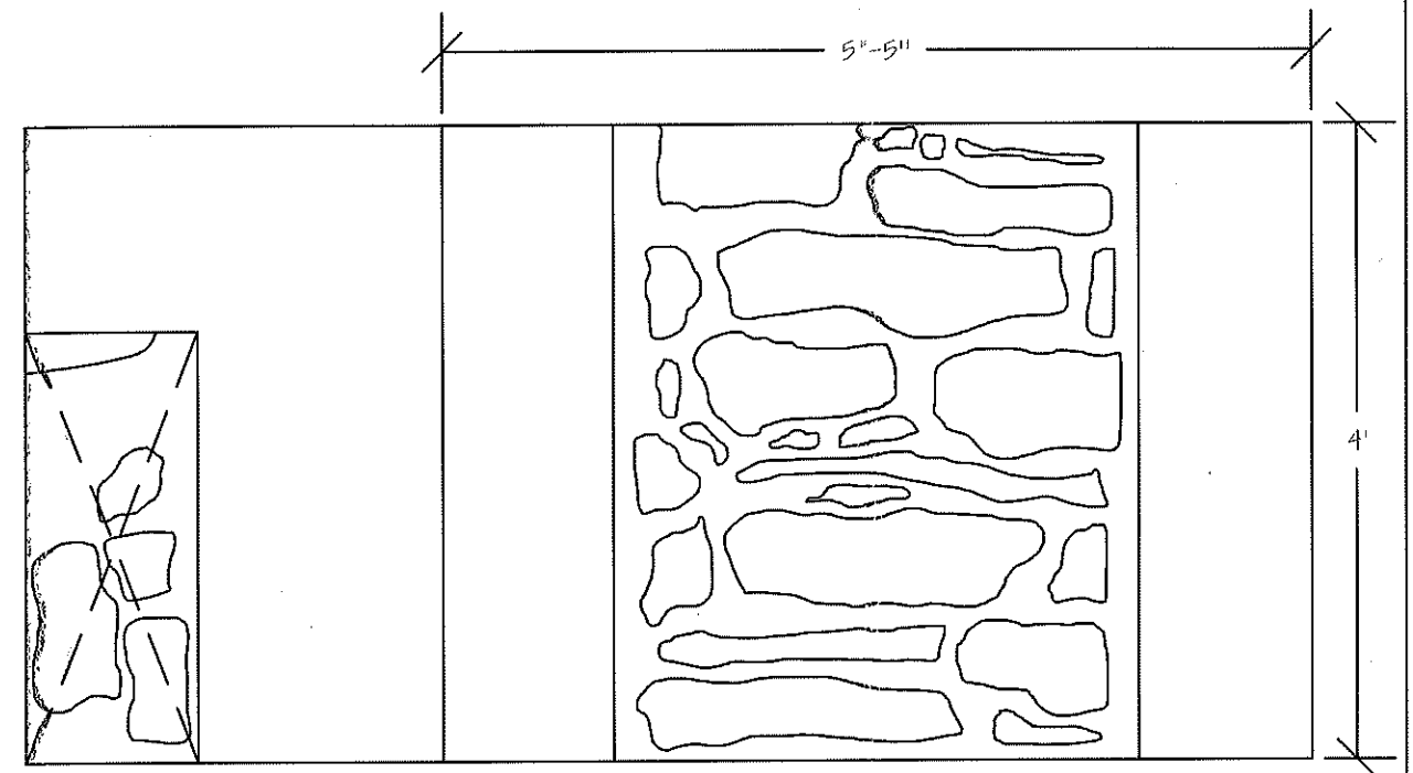
Wall D SR Pivot Wall Scale: 3/4" = 1'-0"
