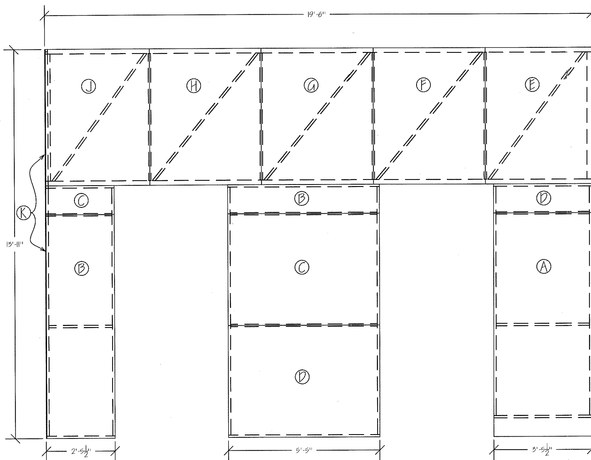
Pivot Wall SL Scale: 1/2" = 1'-0"
