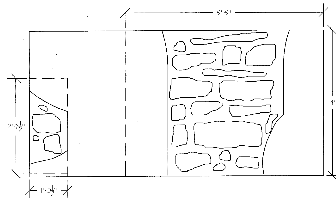
Wall C SL Pivot Wall Scale: 3/4" = 1'-0"
