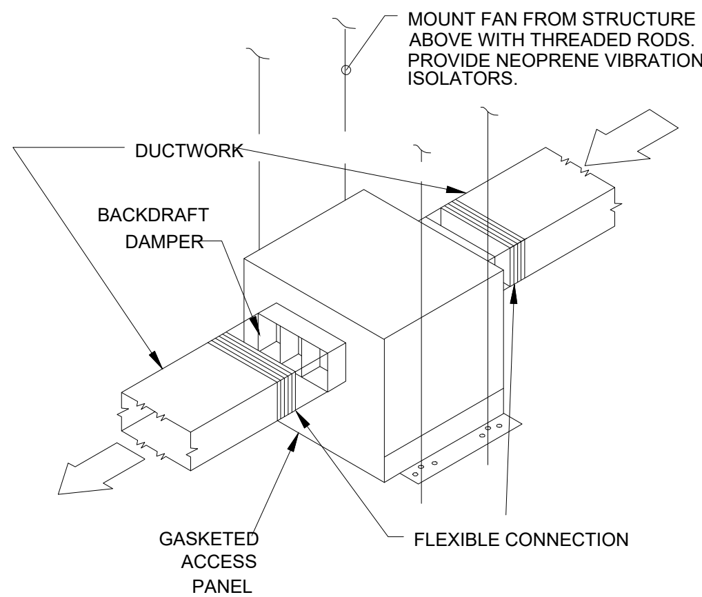
IN-LINE FAN DETAIL
