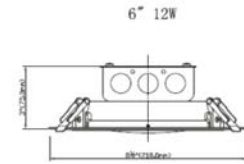
aa: 06 DL06-112WH 120 V 12W 850LM 3000K/4000K
