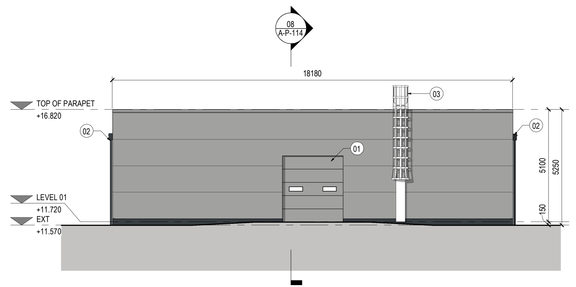
03 FRONT ELEVATION SCALE: 1:100
