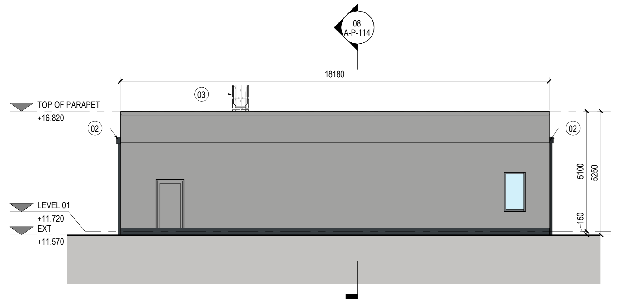
06 REAR ELEVATION SCALE: 1:100
