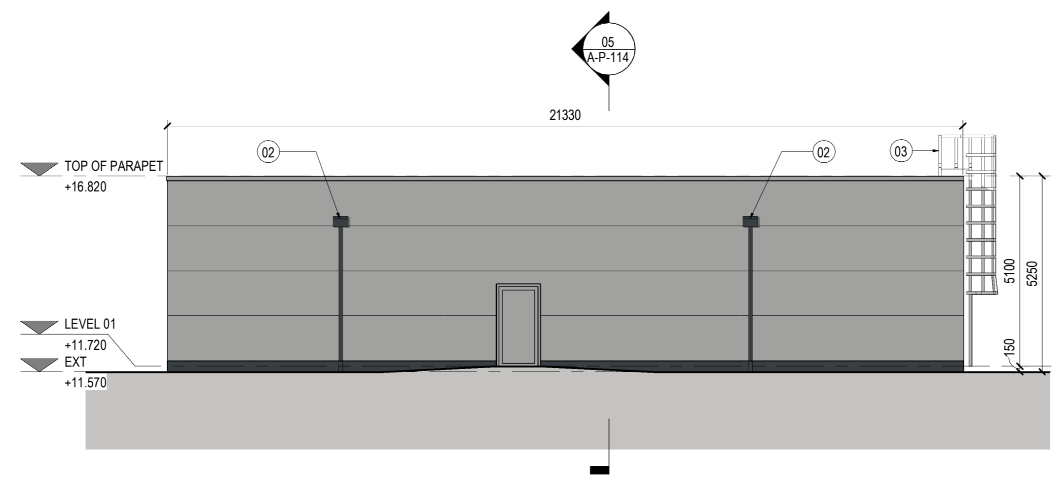
07 LEFT ELEVATION SCALE: 1:100
