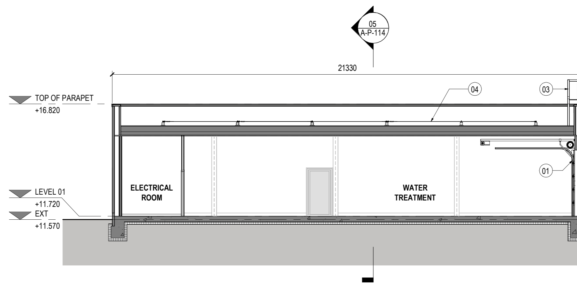
08 SECTION B SCALE: 1:100
