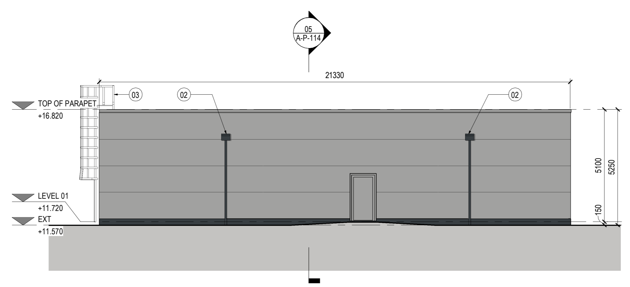
04 RIGHT ELEVATION SCALE: 1:100
