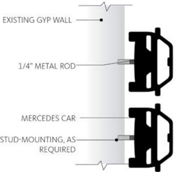
2 SIDE VIEW 3" = 1'-0" A3
