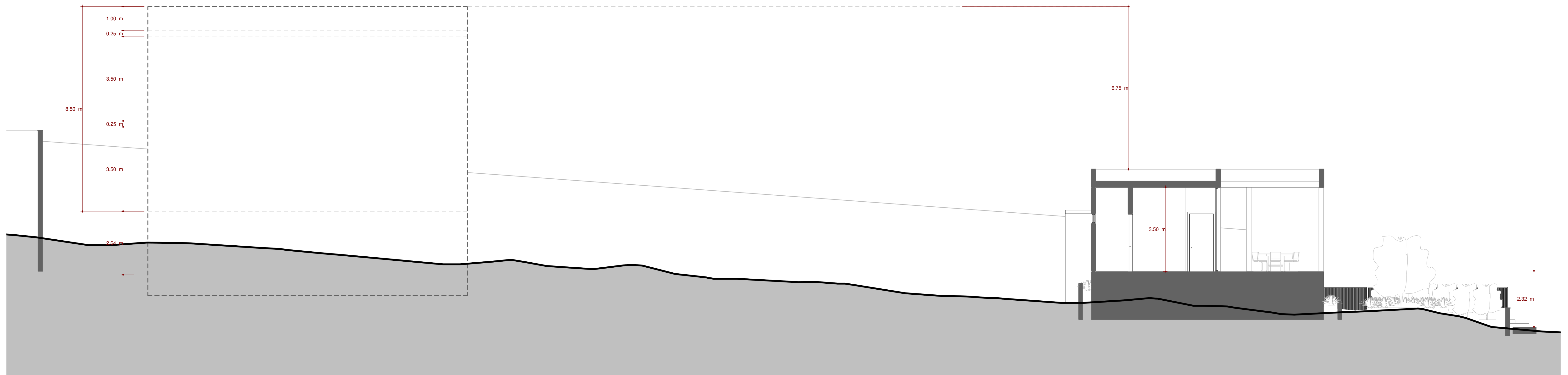
1 Sección 1 : 75
