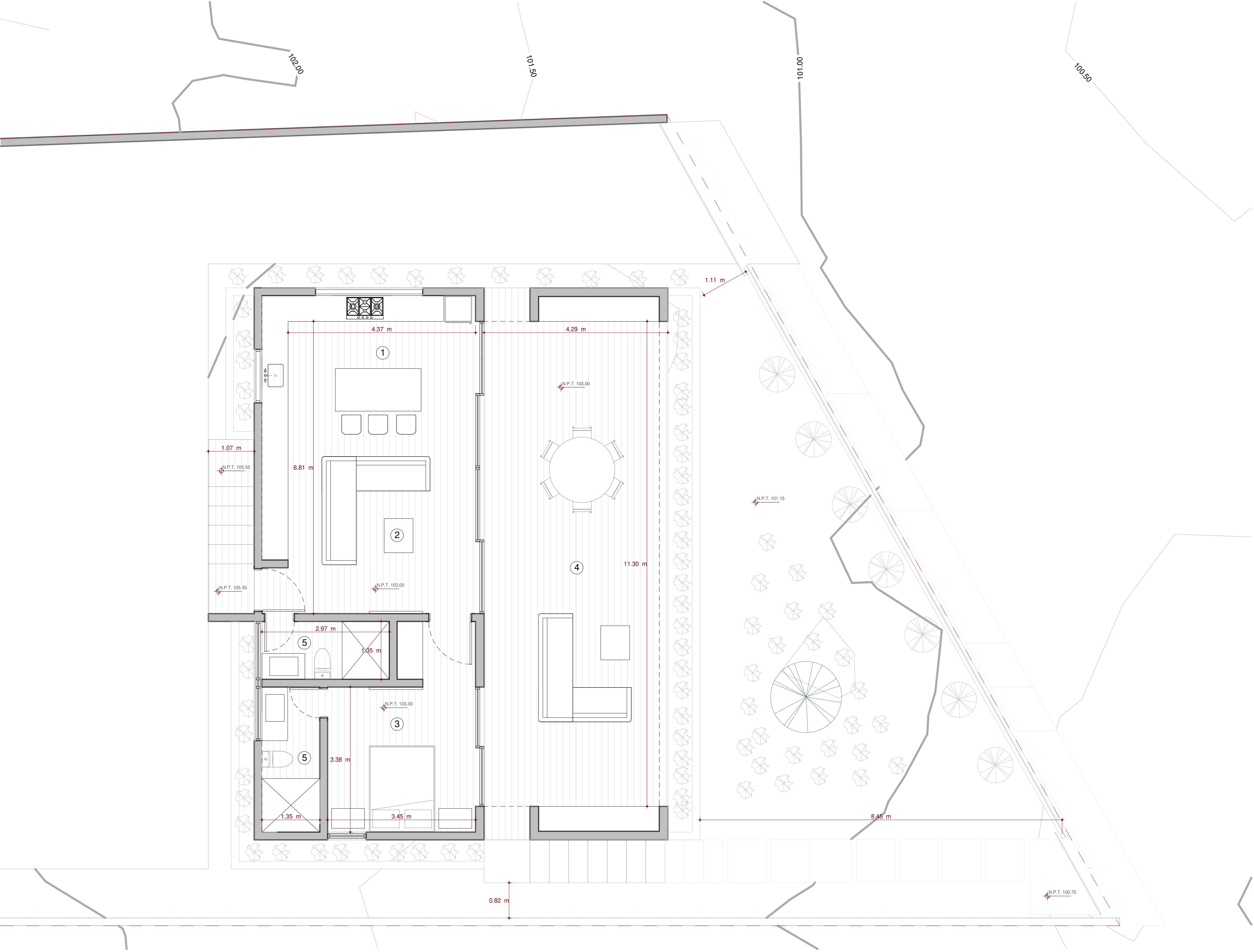
1 Planta Baja 1 : 50
