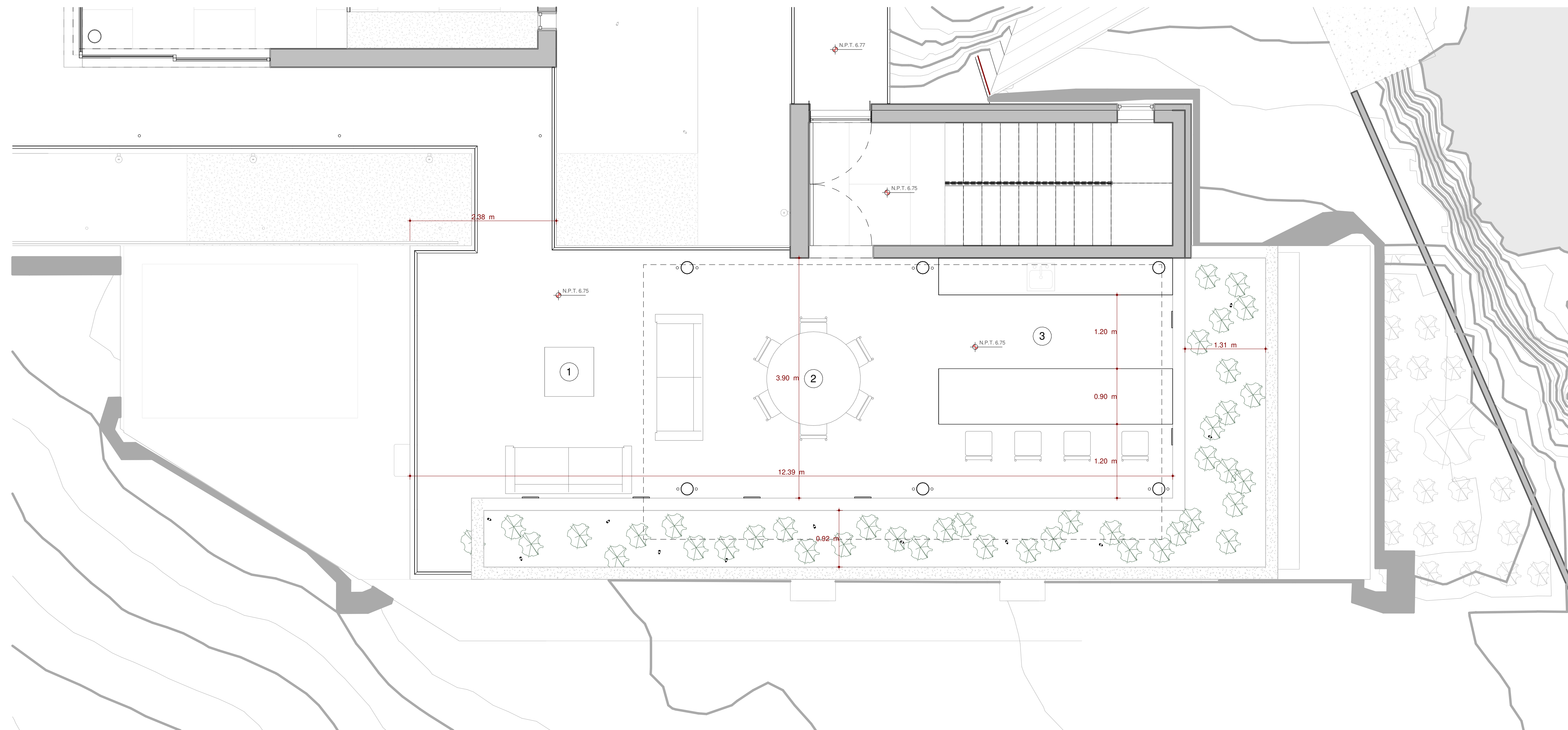
① Level 3 1 : 40
