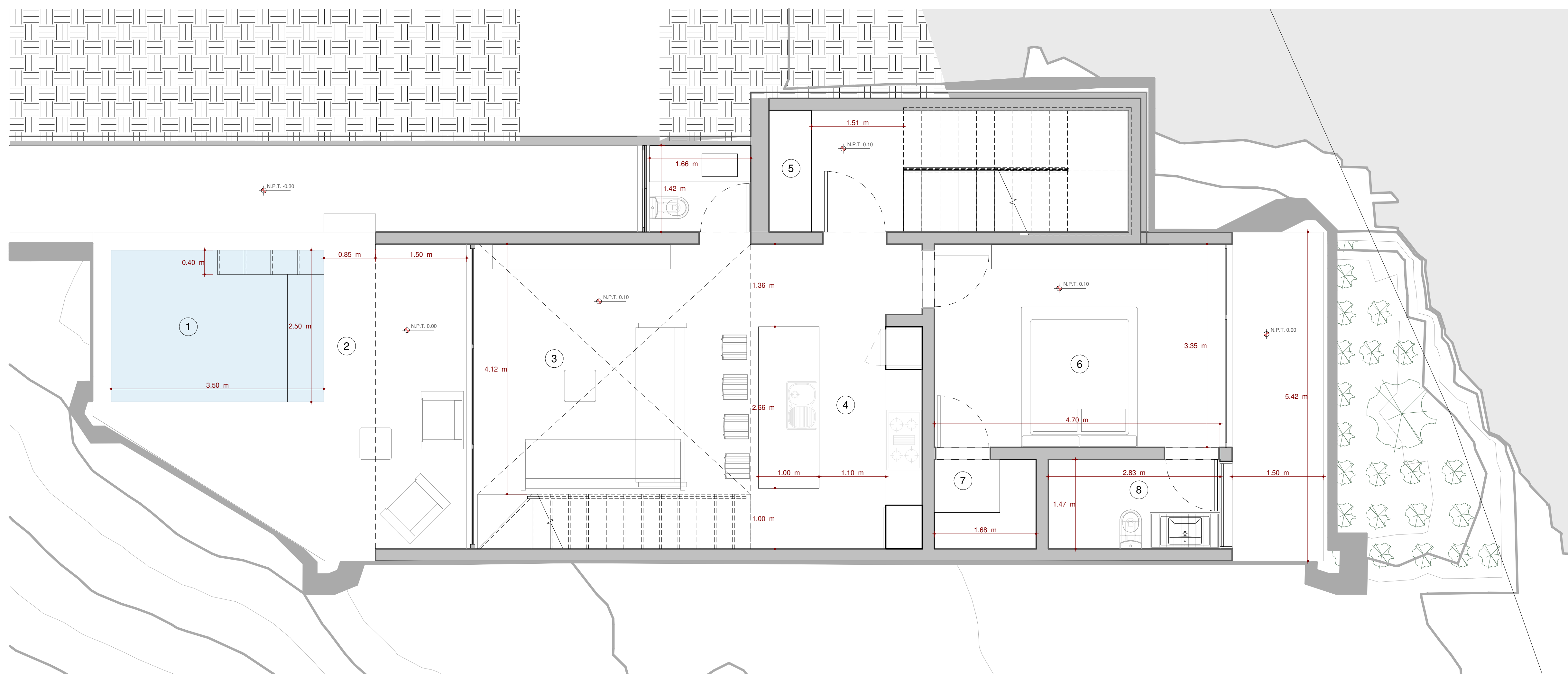
① Level 1 1 : 40
