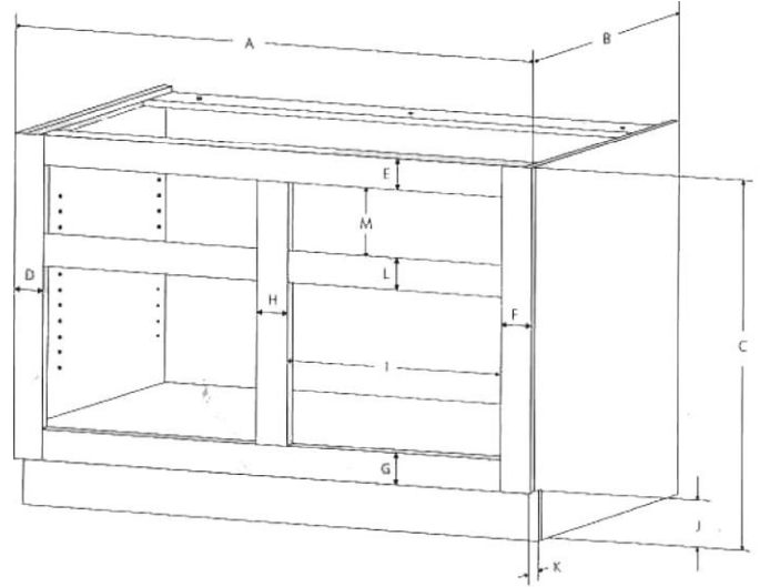
317 | Double Door Base
