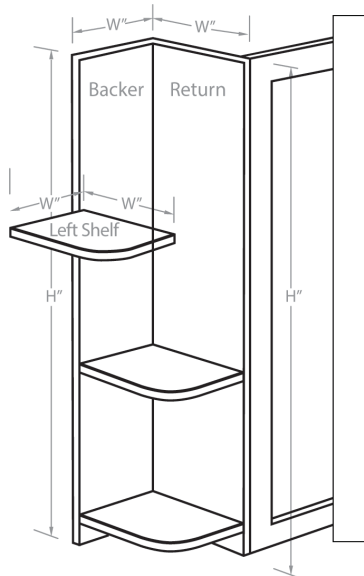
Left Knick Knack Shelf
