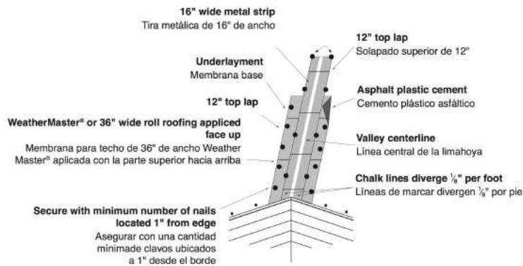
OPEN VALLEY LIMAHOYA DE TIPO VALLE ABIERTO
