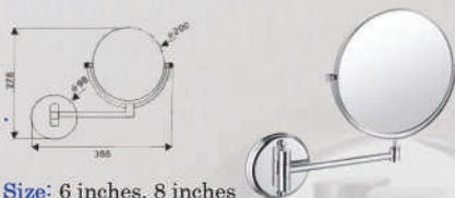
RDH-211-1
