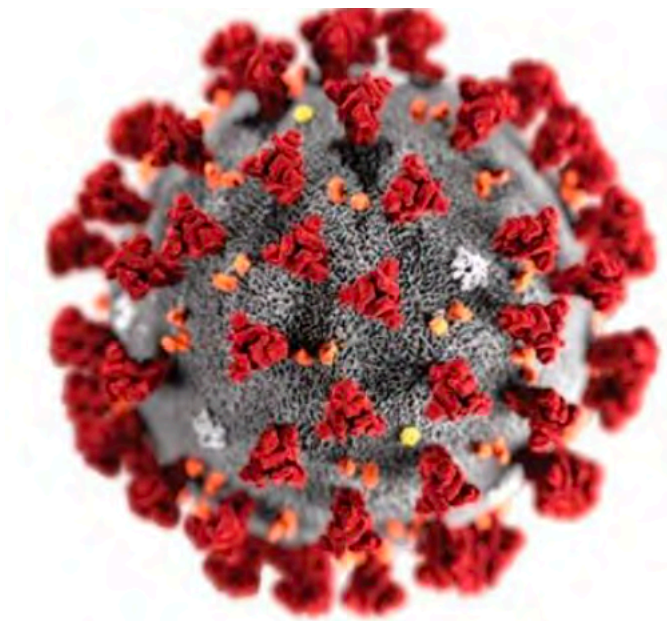
SARS-CoV-2
