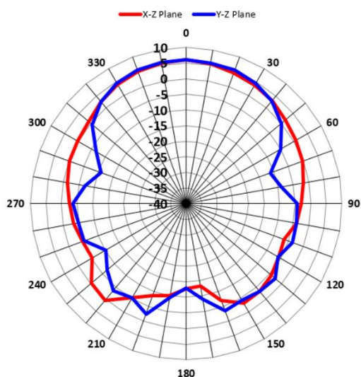
4.5GHz_Horizontal
