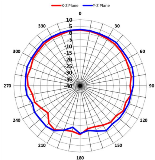
1.8GHz_Horizontal
