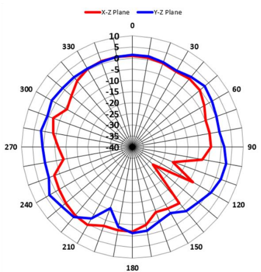
0.9GHz_Horizontal
