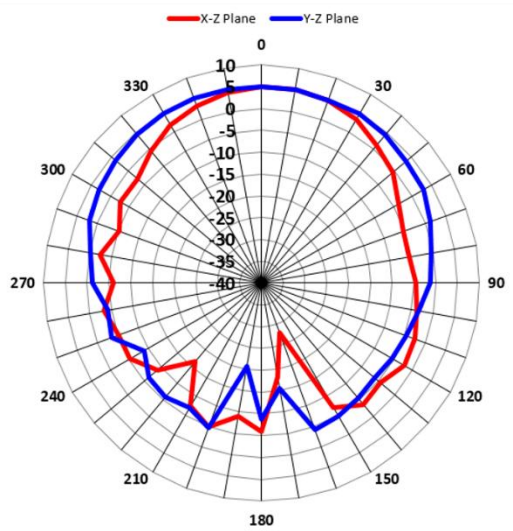
2.4GHz_Horizontal
