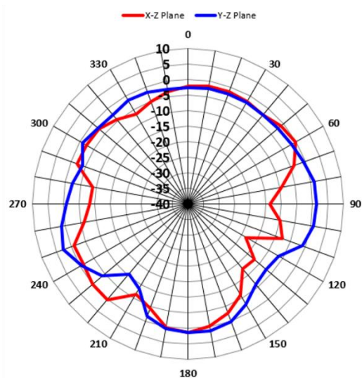
0.7GHz_Horizontal
