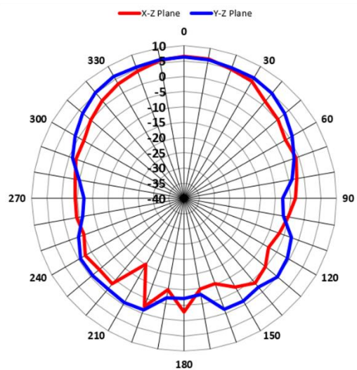
3.5GHz_Horizontal
