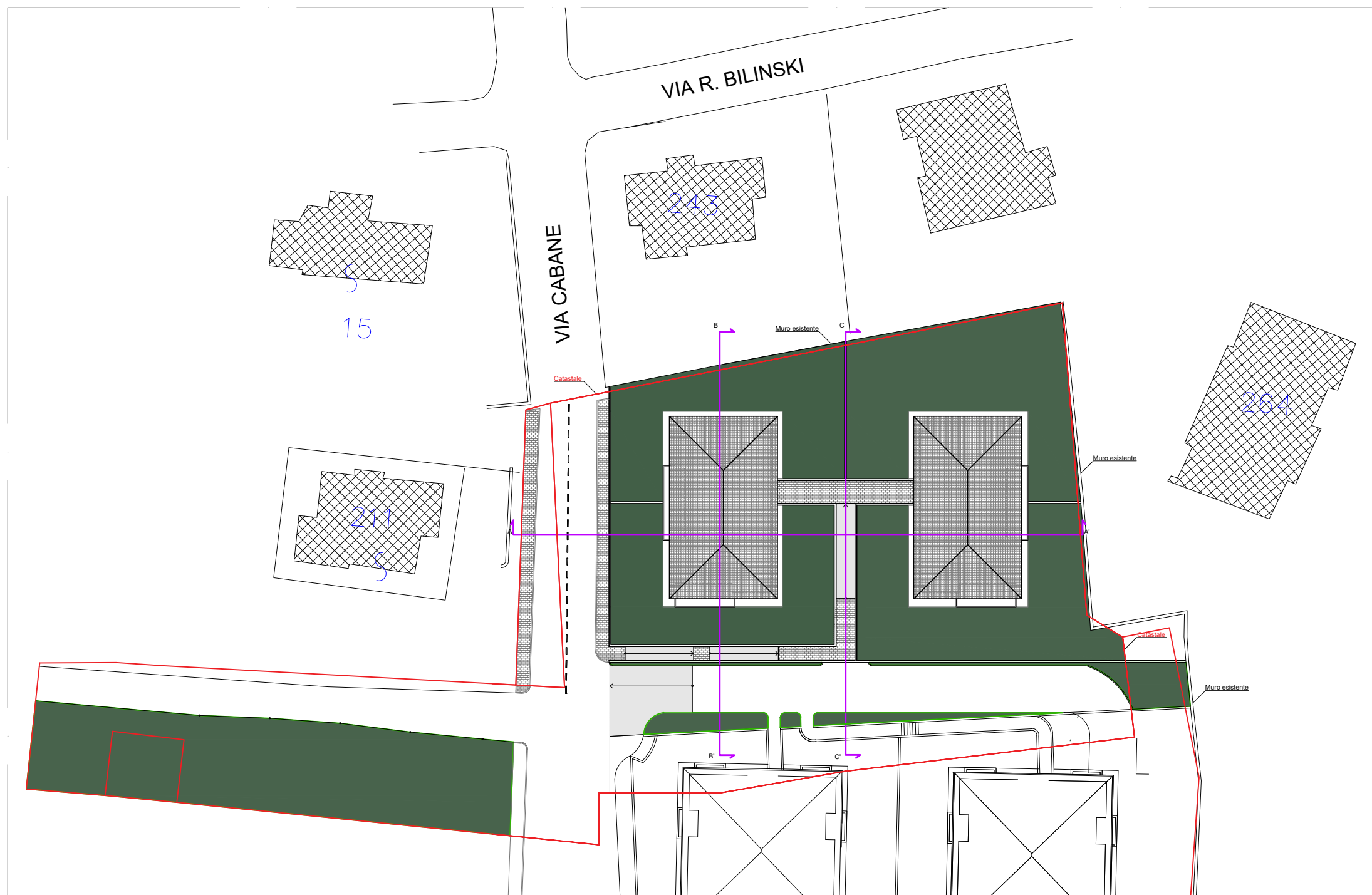
PLANIMETRIA COPERTURE
