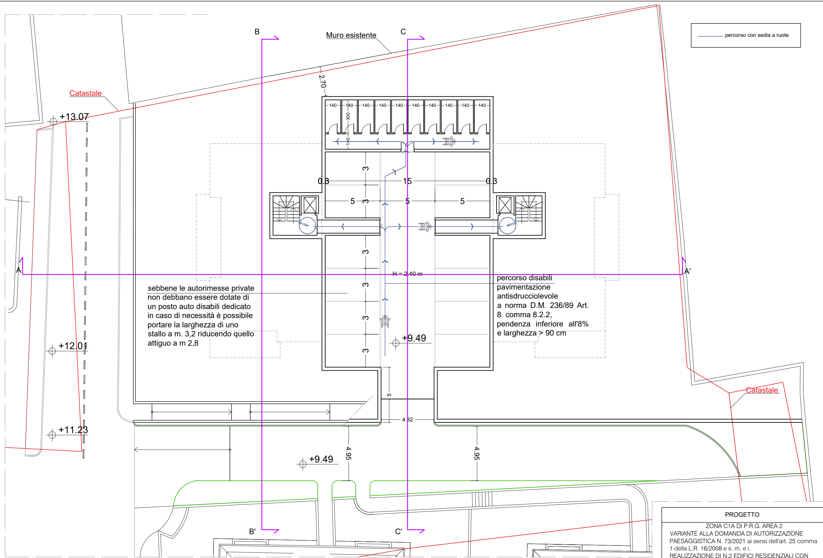
PLANIMETRIA PIANO INTERRATO
