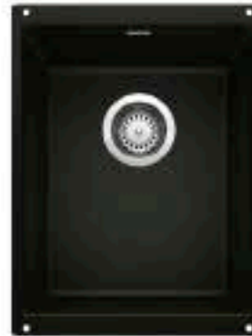
Precis Bar UM OD: 13 3/4" W X 18 1/8" D X 7 15/16" H ID: 12 5/8" W X 15 3/4" D X 7 1/2" H
