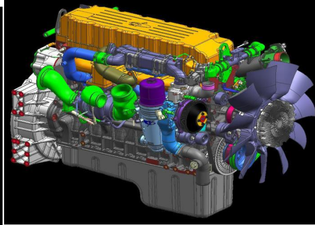
Reference Layout of Engine (Euro 5) Diseño de referencia del motor (Euro 5)
