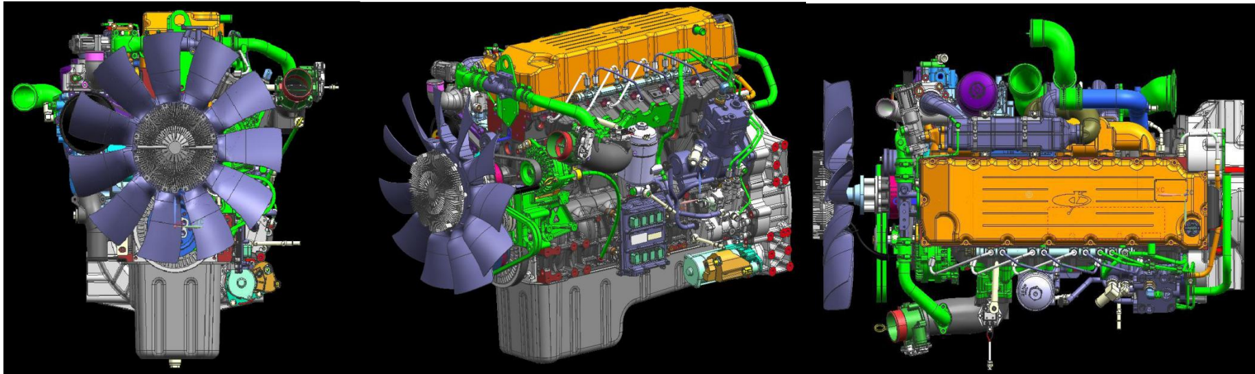
Reference Layout of Engine (Euro 5) Diseño de referencia del motor (Euro 5)
