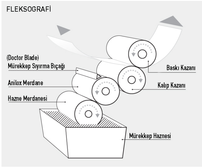
Görsel 9. Fleksografi
