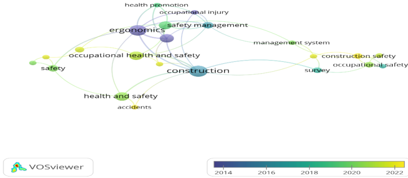
Şekil 3. Anahtar Kelimelerin Yıllara Göre Değişimi
