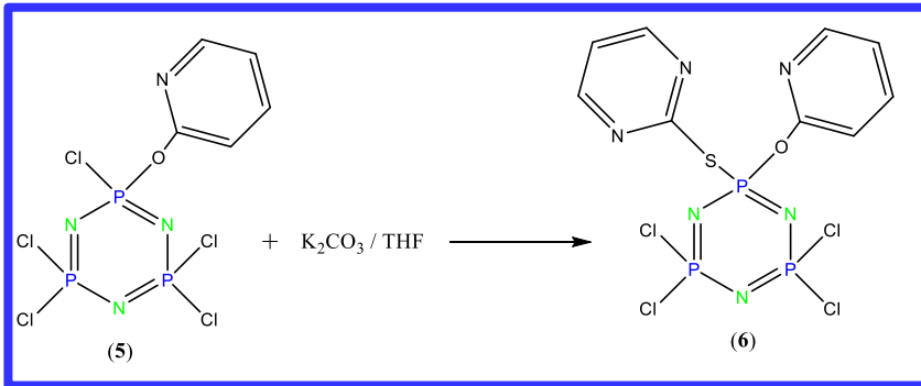
Şekil.4 (6) Bileşiğinin sentezi
