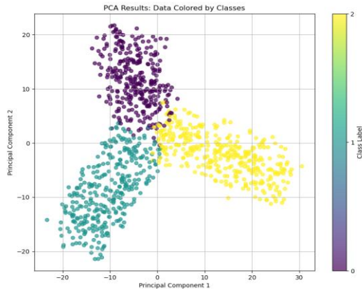
Figure 12. PCA
