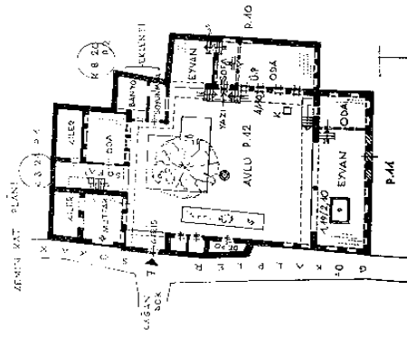
Şekil 5. Günümüzdeki Ziya Gökalp Evinin (Harem Bölümünün) Planı (Tuncer, 1999)
