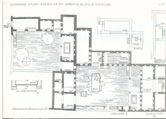
Şekil 4. İlk Olarak Doğan Erginbaş tarafından çizilen yapı planı (Erginbaş, 1954)
