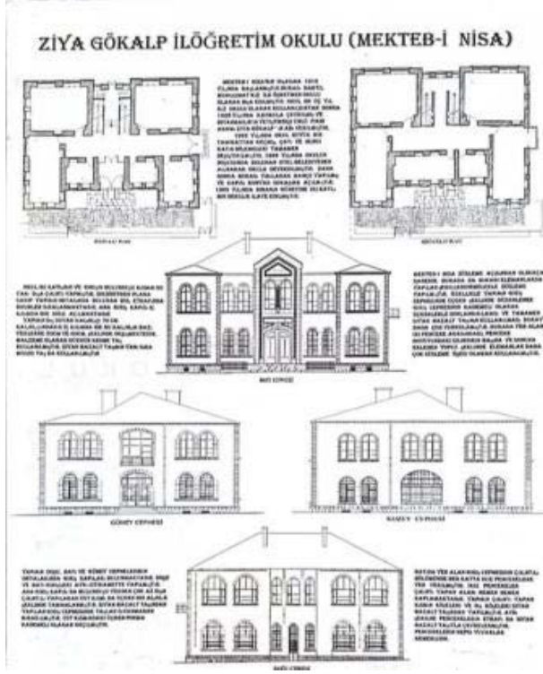
Şekil 12. Ziya Gökalp İlkokulunun Mimari Projesi (Baydaş, 2007).
