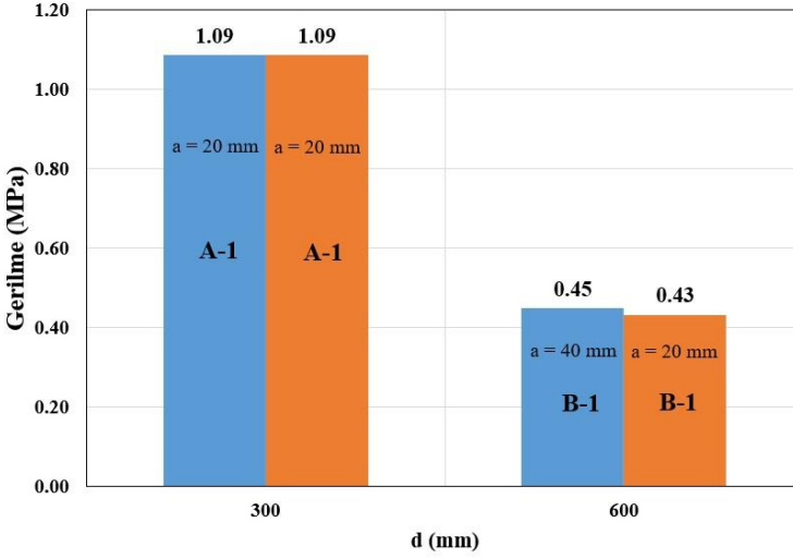
Şekil 5. Maksimum agrega çapı ve boyut etkisi
