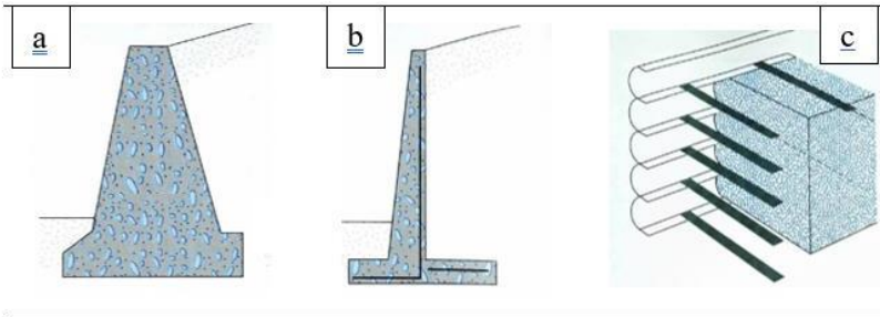
Şekil 1. Dayanma Yapıları: a) Ağırlıklı İstinat Duvarı b) Konsol İstinat Duvarı c) MSE Duvarı (Das, 2011).
