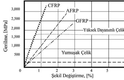
Şekil 1. FRP ve donatılara ait Gerilme-Şekil Değiştirmelerinin karşılaştırılması (Oprisan vd., 2010)
