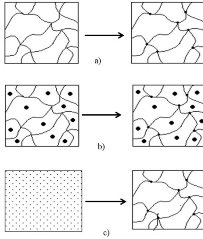
Şekil 2. Çapraz bağlı polimerlerin sentezinde görülebilen durumlar: a) Katı bir polimerin çapraz bağlanması. b) Çözelti halindeki bir polimerin çapraz bağlanması. c) İki monomerin birlikte kopolimerleşmesi ve aynı zamanda da çapraz bağlanması. (Monomerlerden birisi çapraz bağlayıcı olarak davranabilmektedir)
