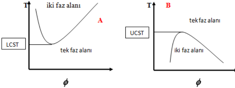
Şekil 1. Sıcaklığa karşı polimer hacim oranı ( \phi ). Polimer çözeltileri için faz diyagramlarının şematik gösterimi: (a) alt kritik çözelti sıcaklığı (LCST) davranışı ve (b) üst kritik çözelti sıcaklığı (UCST) davranışı. (Ward ve Georgiou, 2011; Zhang, J, vd. 2013).
