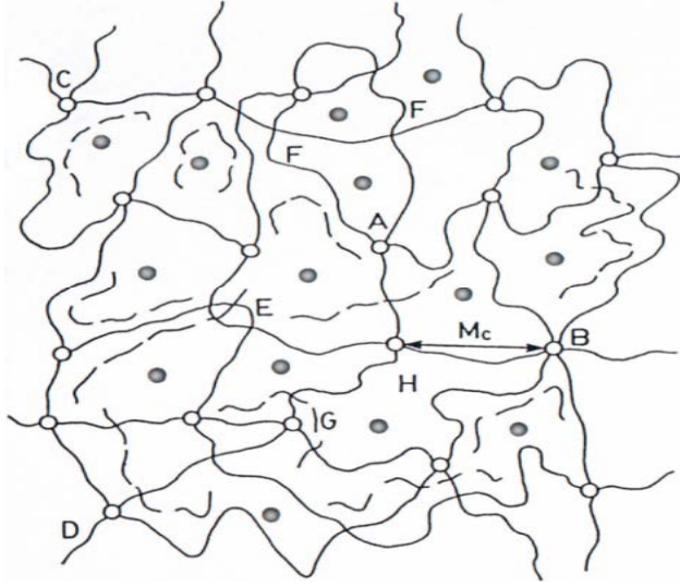
řekil 1. apraz baęlı hidrojelin yapısı. A; Drt fonksiyonlu, B; ok fonksiyonlu apraz baęları gstermektedir. C ve D; Zincir ularıdır. E; Dolařmıř ve birbirine karıřmıř zincirleri gstermektedir. F; İki zincir takılmasını gstermektedir. G; apraz baęlanmamıř kk zincirleri gsterir. Mc; İki apraz baę merkezi arasındaki zincirin molekl ktlesidir. H; difzlenme iin uygun olan apraz baęlar arasındaki bořluk. •; apraz baęlar arasındaki bořluklara difzlenen zc
