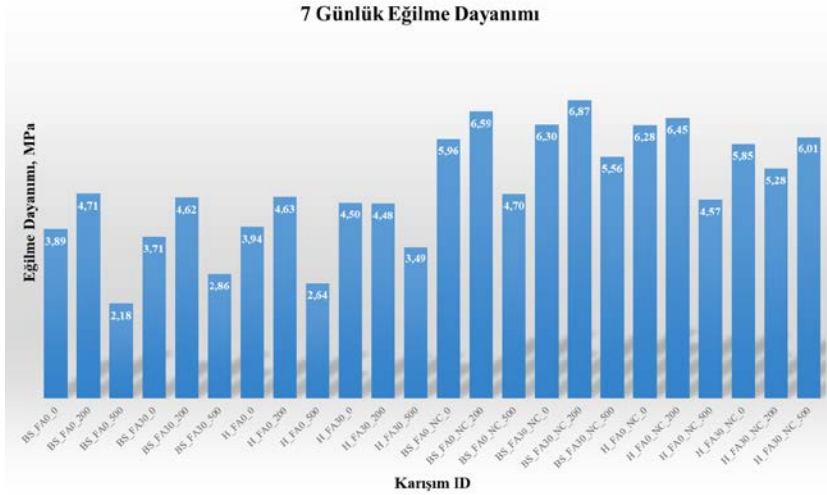
Şekil 4.7. 7 günlük kür yaşı eğilme dayanımı değerleri.
