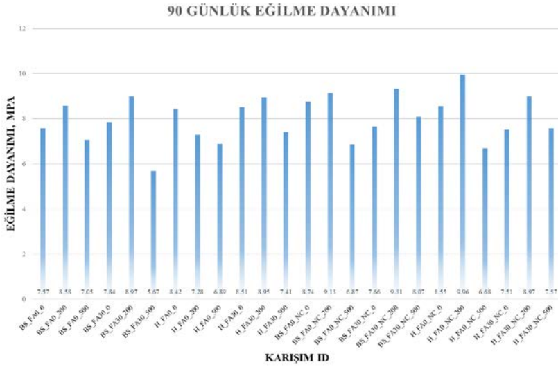
Şekil 4.20. günlük kür yaşı eğilme dayanımı değerleri.
