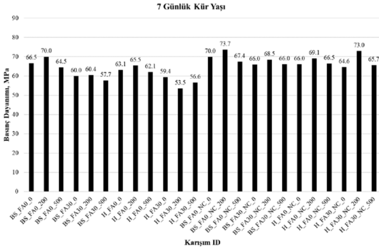
Şekil 4.1. 7 günlük kür yaşı basınç dayanımı değerleri.
