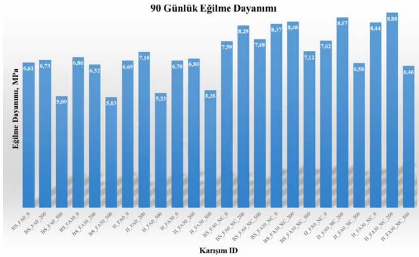
Şekil 4.9. 90 günlük kür yaşı eğilme dayanımı değerleri.
