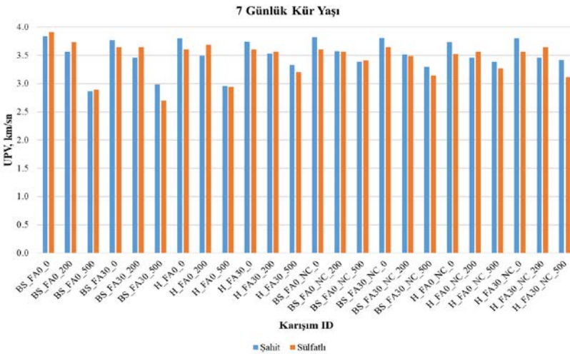
Şekil 4.15. 7 günlük kür yaşı UPV değerleri.
