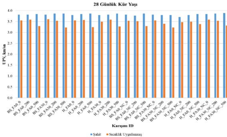
Şekil 4.5. 28 günlük kür yaşı UPV değerleri
