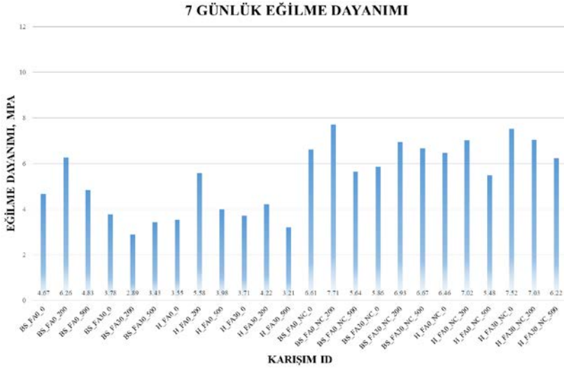
Şekil 4.18. 7 günlük kür yaşı eğilme dayanımı değerleri.
