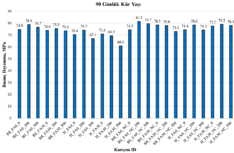
Şekil 4.12. 90 günlük kür yaşı basınç dayanımı değerleri.
