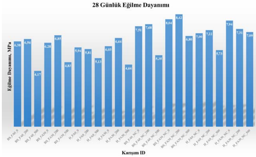
Şekil 4.8. 28 günlük kür yaşı eğilme dayanımı değerleri.
