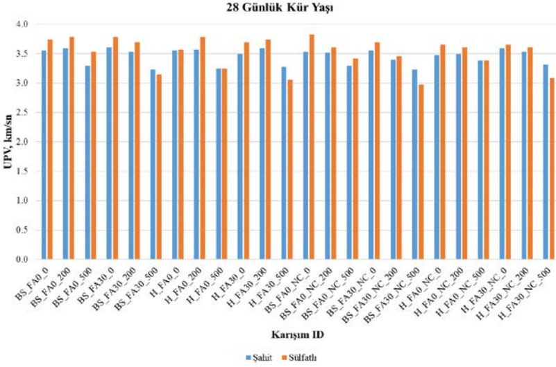
Şekil 4.16. 28 Günlük Kür Yaşı UPV Değerleri
