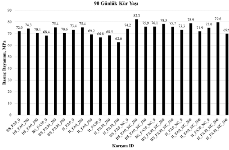
Şekil 4.3. 90 günlük kür yaşı basınç dayanımı değerleri.
