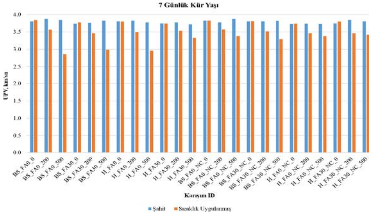
Şekil 4.4. 7 günlük kür yaşı UPV değerleri.
