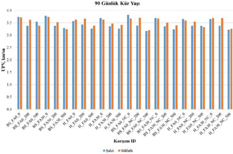
Şekil 4.17. 90 günlük kür yaşı UPV değerleri.
