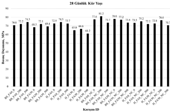
Şekil 4.2. 28 günlük kür yaşı basınç dayanımı değerleri.
