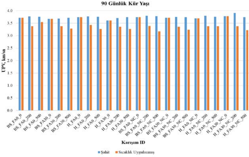
Şekil 4.6. 90 günlük kür yaşı UPV değerleri.
