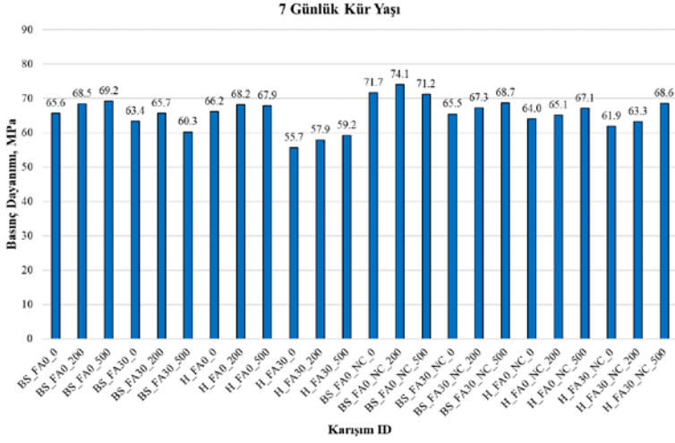
Şekil 4.10. 7 günlük kür yaşı basınç dayanımı değerleri.
