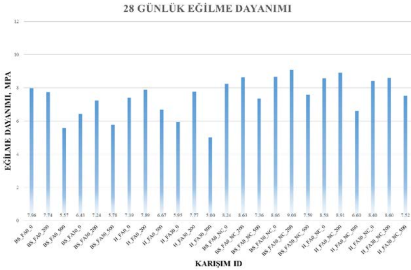
Şekil 4.19. 28 günlük kür yaşı eğilme dayanımı değerleri.
