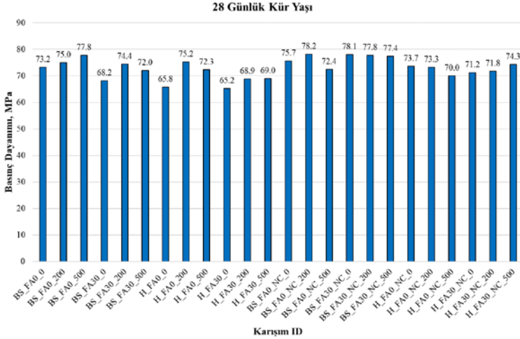
Şekil 4.11. 28 günlük kür yaşı basınç dayanımı değerleri.
