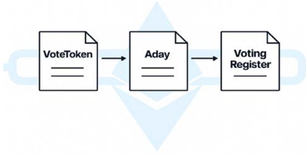
Şekil 2. Akıllı Sözleşmeler
