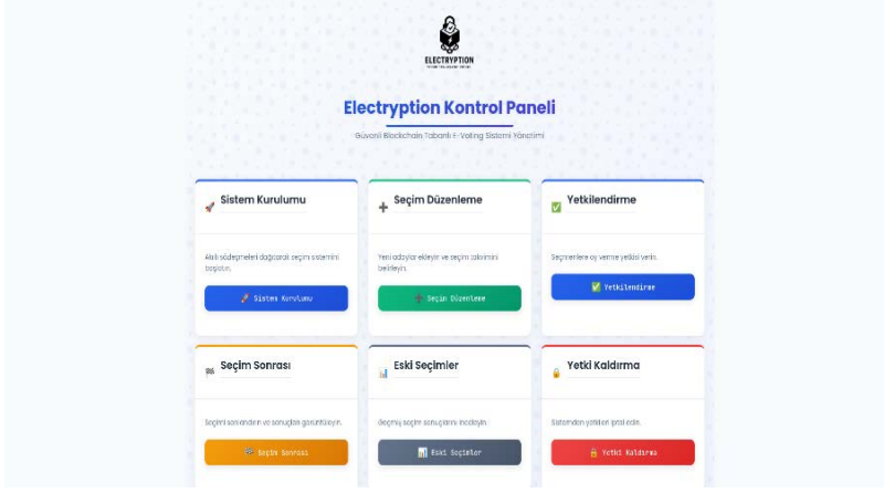
Şekil 4. Kontrol Paneli
