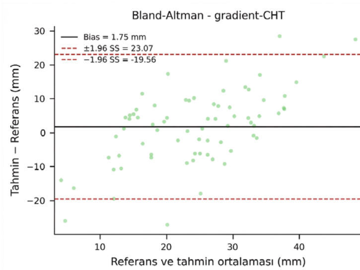
Şekil 5. Bland–Altman grafiği
