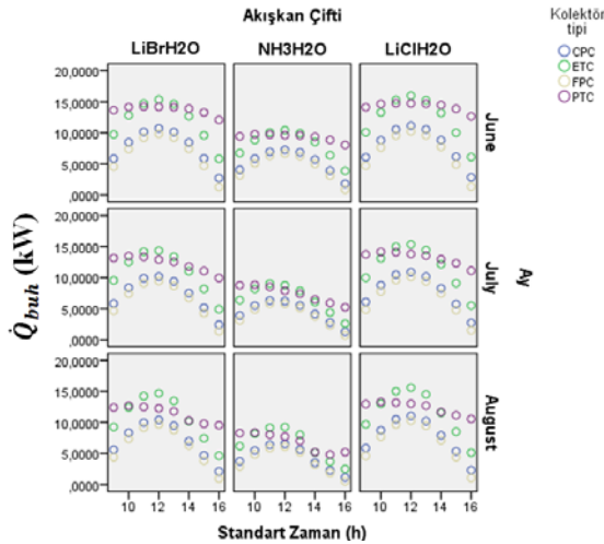
Şekil 6. Buharlaşma ısı geçiş miktarı (soğutma kapasitesi) değişimi
