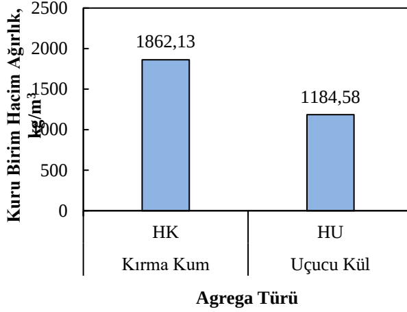
Şekil 1. Agregat türüne göre kuru birim hacim ağırlık.
