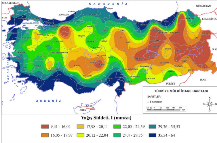
Şekil 1. Yağış şiddeti haritası (5 yıl tekerrür aralıklı, 60 dakika süreli)
