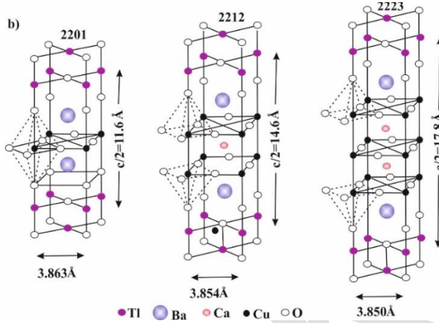
Şekil 6 Tl-bazlı HTS kristal yapıları a) TlBa_2Ca_{n-1}Cu_nO_{2n+3} genel formülü ile verilen seri, b) Tl_2Ba_2Ca_{n-1}Cu_nO_{2n+4} genel formülü ile verilen seri (Schrieffer vd., 2007; Onar,2017).
