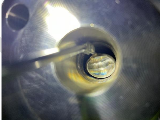
Şekil 2. Boru kök kaynağının ayna yardımı ile yapılan görsel kontrolü
