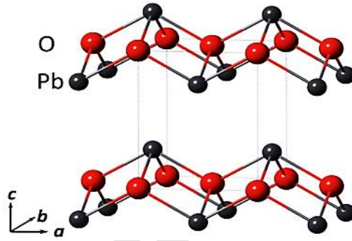
Şekil 12. \text{PbO} 'in kristal yapısı
