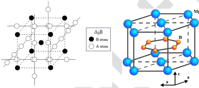
Şekil 1. a) A 3 B bileşiklerinin kristal yapısı (Mourachkine, 2004), b) MgB 2 'nin kristal yapısı
