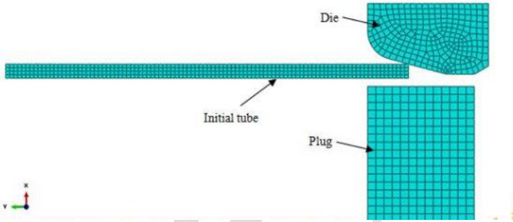
Şekil 2. Boru soğuk çekim prosesi [6]
