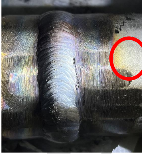
Şekil 1. Görsel muayene sırasında tespit edilen çok küçük yüzeye açık gözenekler.
